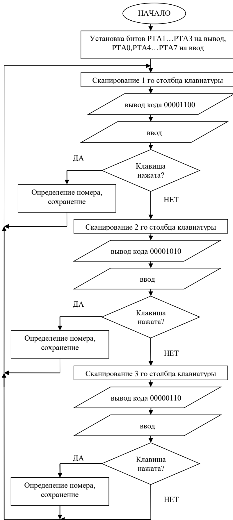
Рисунок 2.6 Блок-схема программы опроса 12-ти кнопочной клавиатуры
