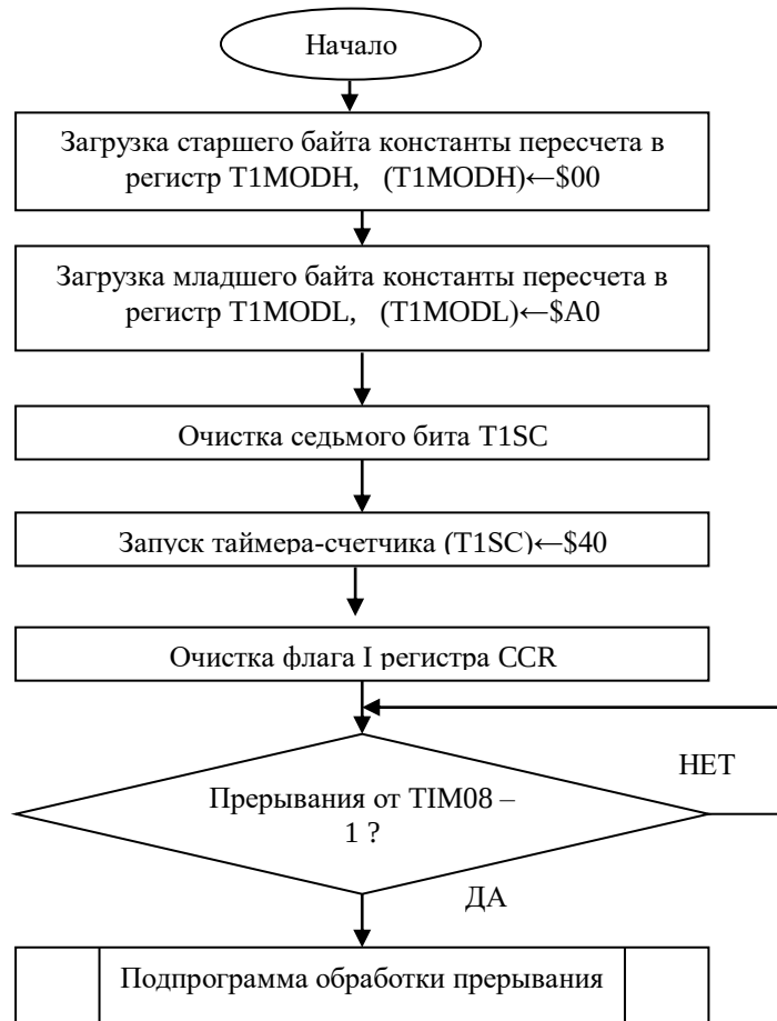
Рисунок 2.8 Блок-схема программы формирования временной задержки 20 мкс в режиме таймера
