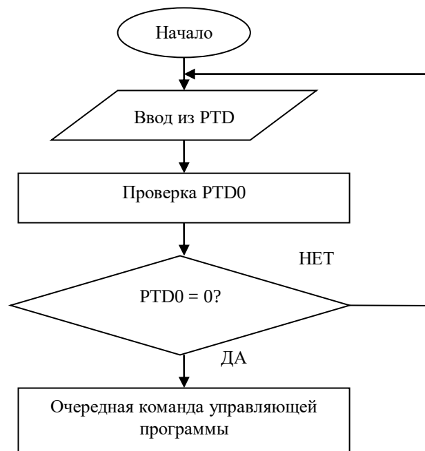
Рисунок 2.4 Блок-схема программы реализации контроля переключения ключа
