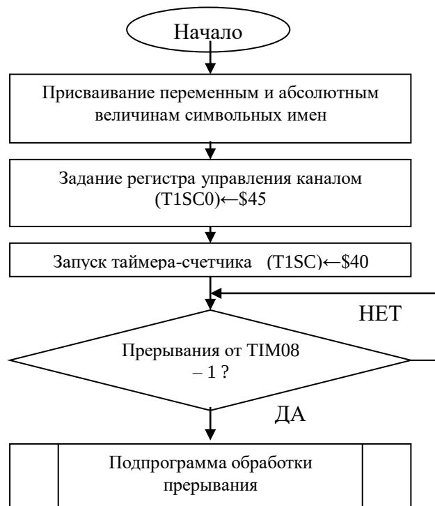
Рисунок 2.11 Блок-схема программы реализации режима захвата таймерного модуля TIM08 при положительном переходе сигнала
