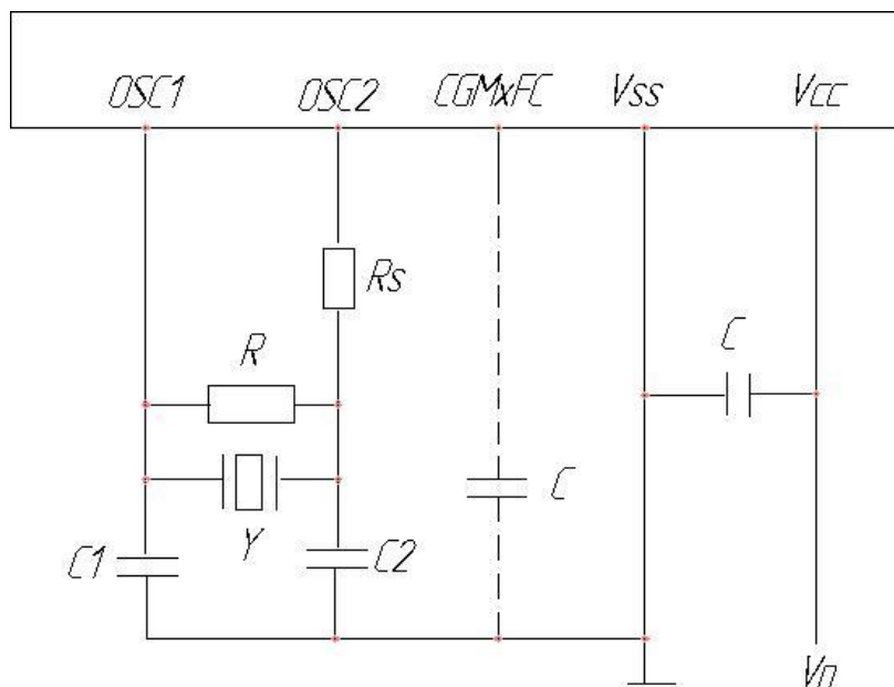
Рисунок 1.4 Схема подключения кварцевого резонатора
