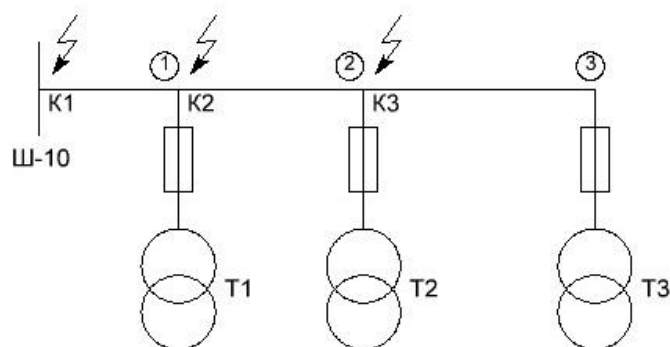
Рис. 3 Расчетная схема сети 10 кВ
