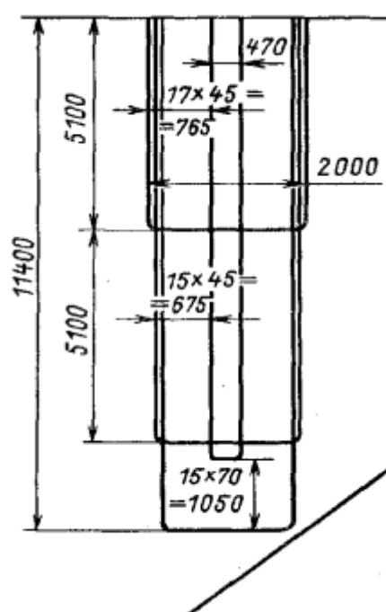
Рис. Размеры секции ширмового пароперегревателя
