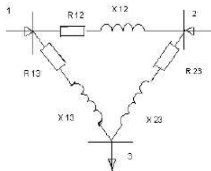
Рис.2. Схема замещения сети из трех узлов с активно-индуктивными связями
