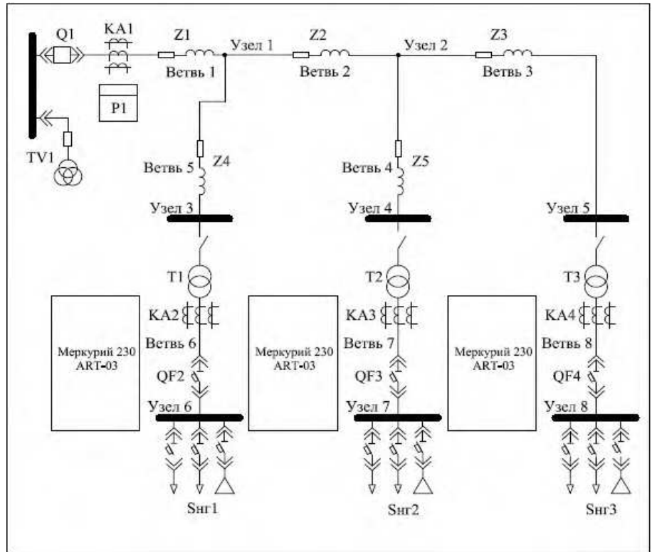
Рис. 2. Электрическая схема исследуемого участка сети
