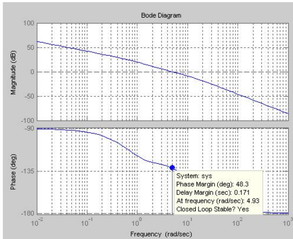
Рис. 3.6. ЛЧХ контура скорости с астатизмом первого порядка
