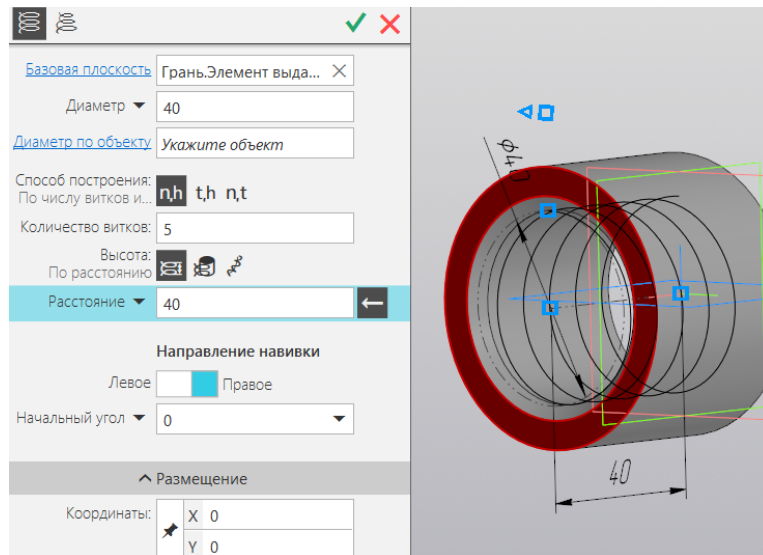
Рис. 6 – Спираль в отверстии втулки
