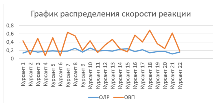
Рис. 2 – График распределения скорости реакции
