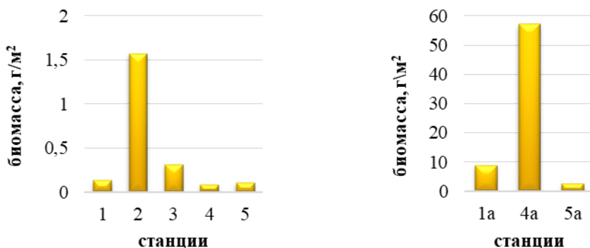
Рис.11. Биомасса (г/м 3 ) мягкого зообентоса в районе водозабора Зай ГРЭС Fig. 11. Biomass (g/m 3 ) of soft zoobenthos in the water intake area of Zai SDPP
