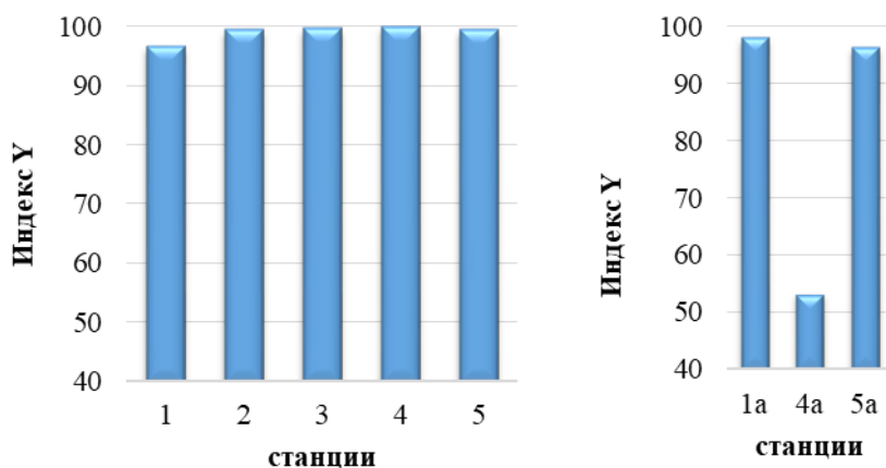
Рис. 23. Индексы состояния донного гидробиоценоза Y в районе водозабора ЗайГРЭС Fig. 23. Indices of the state of benthic hydrobiocenosis Y in the water intake area of Zai SDPP
