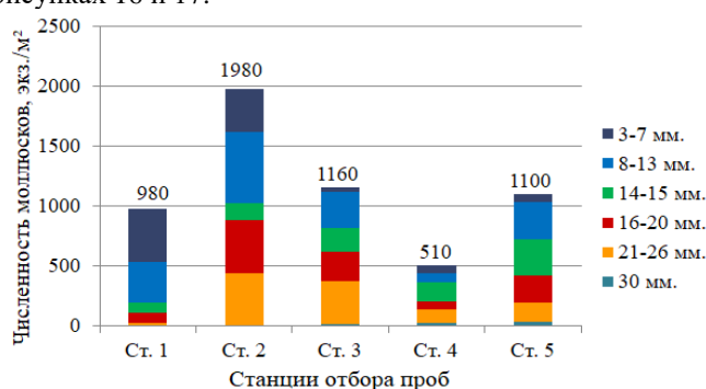
Рис.16. Численность D. polymorpha в районе Fig.16. Abundance of D. polymorpha in the water водозабора Зай ГРЭС intake area of Zai SDPP
