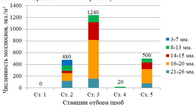
Рис.17. Численность D. bugensis в районе Fig.17. Abundance of D. bugensis in the water intake водозабора Зай ГРЭС area of Zai SDPP
