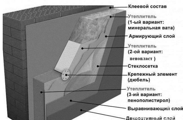
Рисунок 2. Устройство фасадной теплоизоляционной системы с тонким штукатурным слоем
