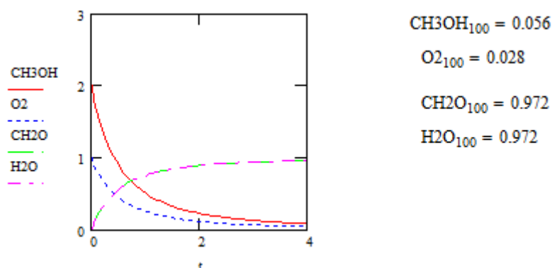
Рис. 4. Общая модель реактора РИВ
