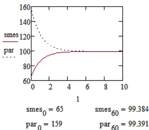
Рис. 2. Модельный эксперимент теплообменника
