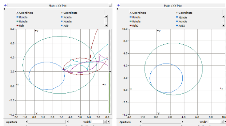
Рис. 3. Характеристики срабатывания реле сопротивления дистанционной защиты, уставки без учета РГ (слева – Д31, справа – Д32)
