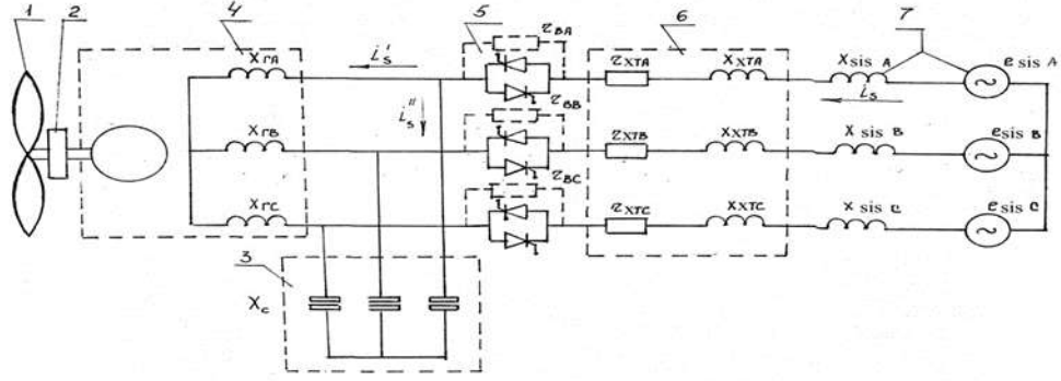
Рис. Схема ветряной электрической установки
