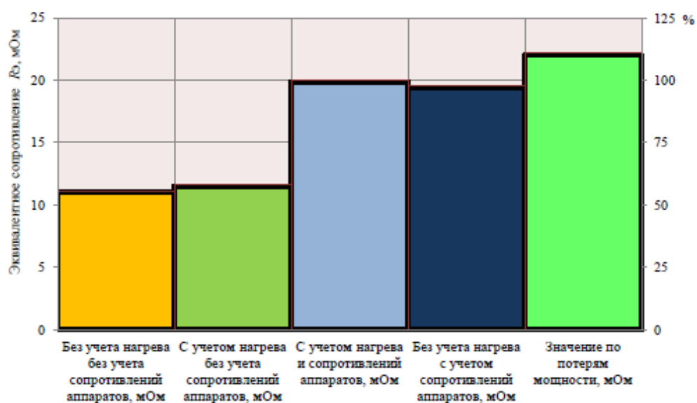
Рис. 3. Возможная вариация эквивалентного сопротивления схемы
