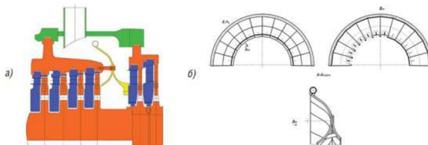
Рис. 3. Кольцевая камера для подвода контура НД в турбине Т-53/67-8.0:
