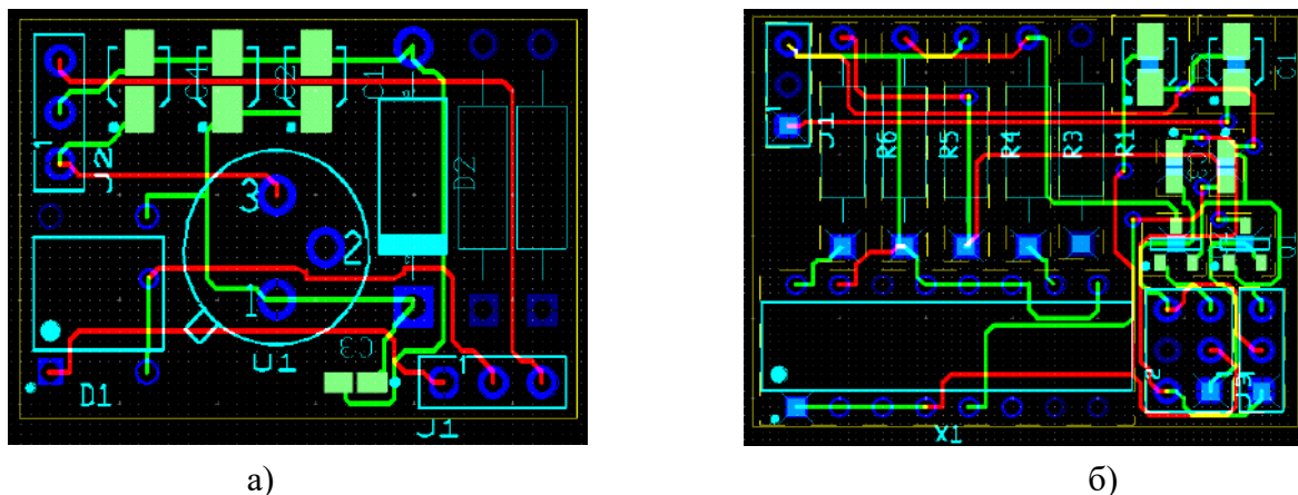
Рис. 1. Трассировка печатных плат, а) обработки информации, б) инвертора
