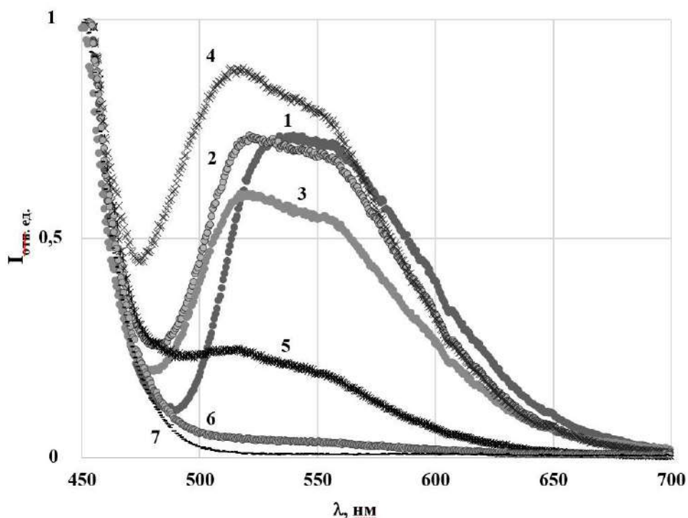
Рис. 2. Спектры люминесценции образцов ИАГГ:Се керамики с разным соотношением Al/Ga : 1- 5/0, 2 - 4/1, 3- 4/1, 4 - 3/2, 5 – 2/3, 6 – 1/4, 7 - 0/5
