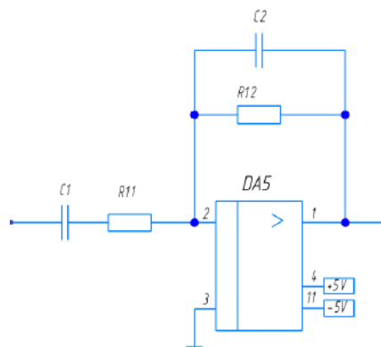
Рис.5 Интегратор
