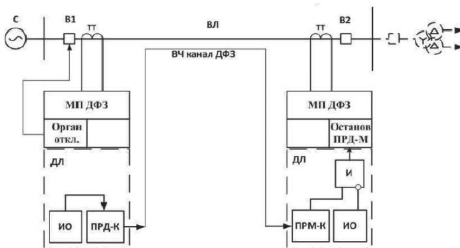
Рис. 1. Структурная схема ДФЗ
