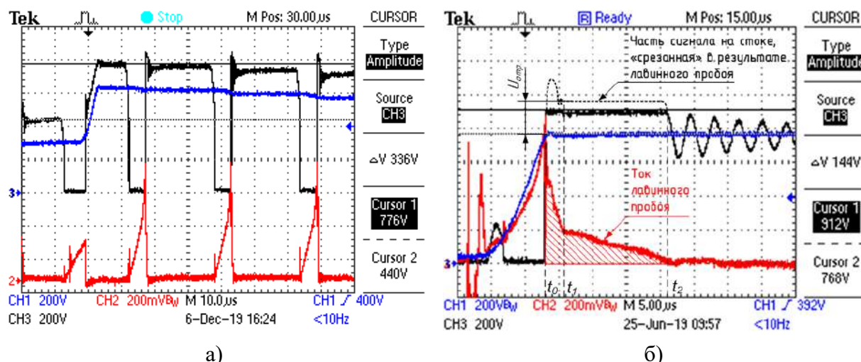
Рис. 1. Осциллограммы процессов в ОПККМ в момент воздействия помехи
