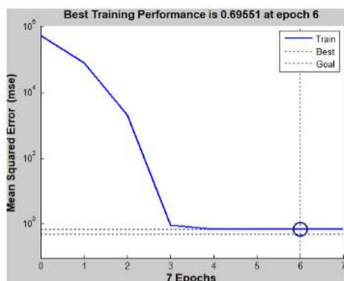
Рис.2. Изменение среднеквадратичной ошибки нейронной сети в процессе обучения
