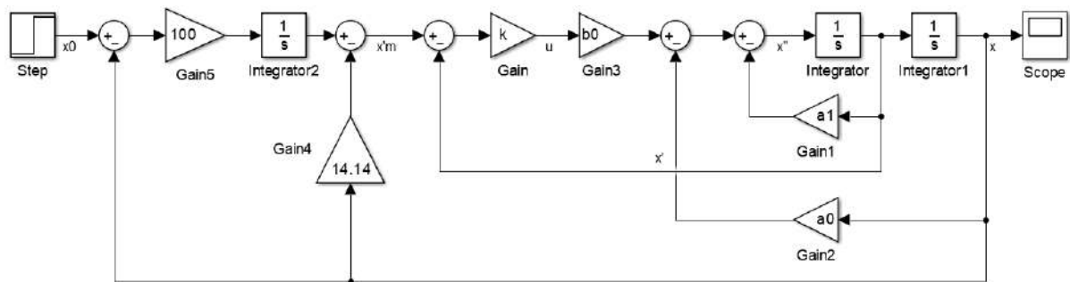
Рис. 1. Simulink-модель электромеханической системы с компенсационным алгоритмом управления
