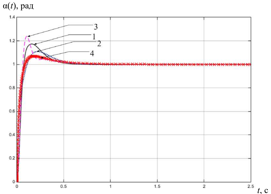
Рис. 1 Переходные характеристики системы
