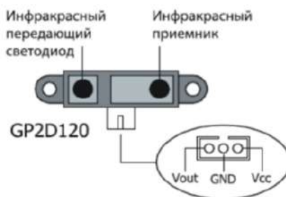
Рис. 2. Инфракрасный измеритель расстояния GP2D120
