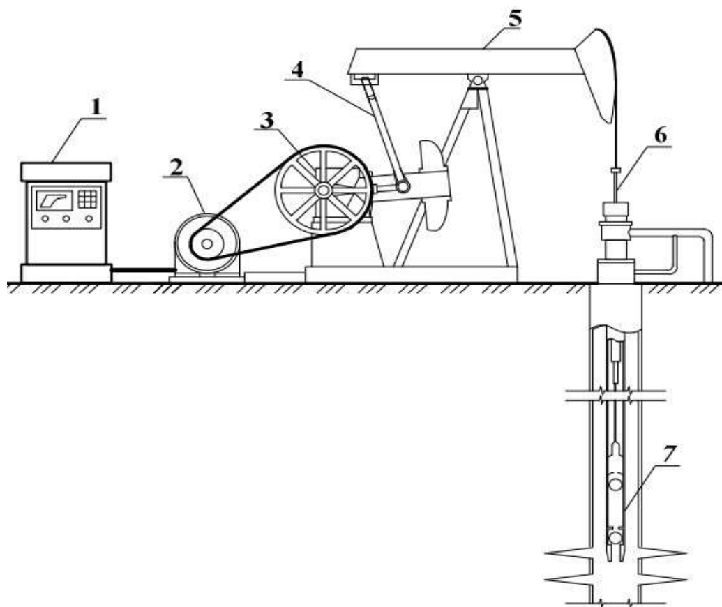
Упрощенная схема установки СШН
