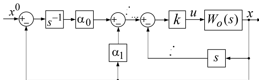
Рис. 2. Структурная схема электромеханической системы при нулевых начальных условиях
