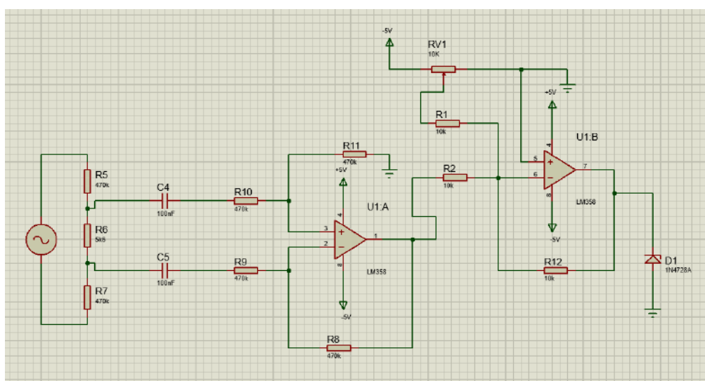
Рис. 2 Вариант схемы измерителя TrueRMS значений в ProteusISIS
