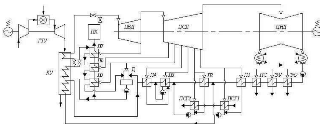
Рис. 2. Принципиальная тепловая схема ПГУ с параллельной схемой работы ПК и КУ с паровой турбиной Т-100/120-130
