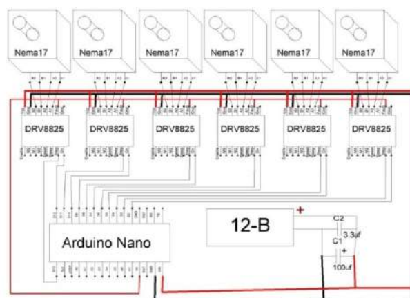
Рис.3. Принципиальная схема электрической части разрабатываемого робота манипулятора
