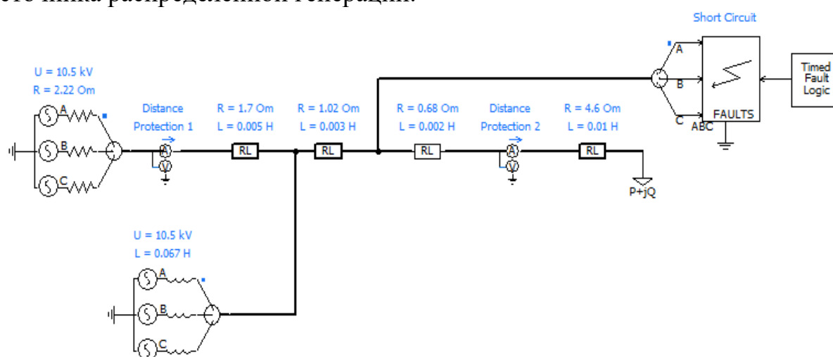
Рис. 2. Модель участка сети в программном комплексе PSCAD/EMTDC
