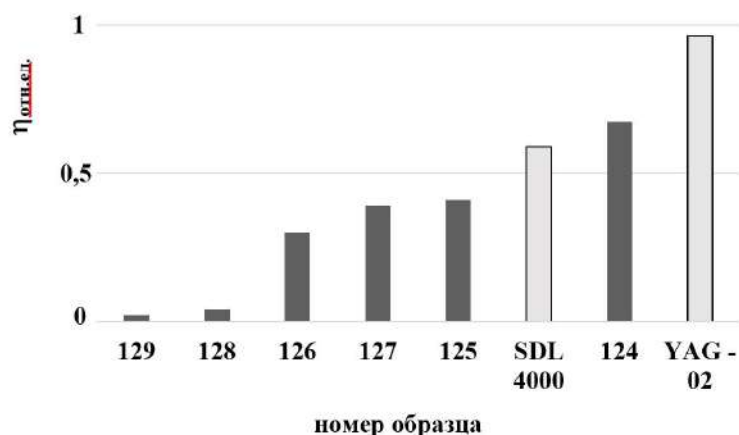
Рис. 3. Относительные эффективности преобразования излучения чипа люминофорами
