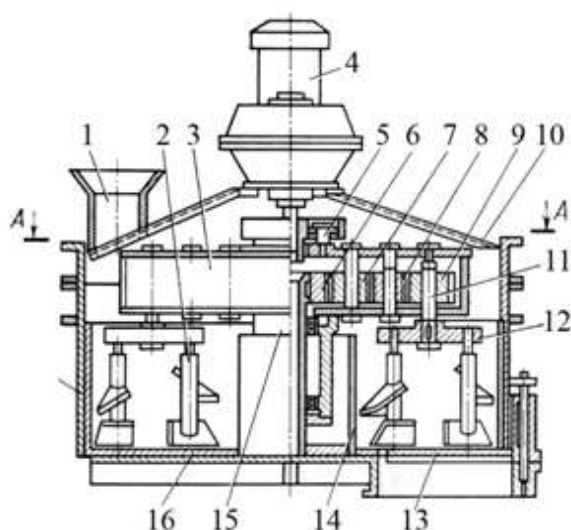
Рис. 1. Технологическая схема бетоносмесителя
