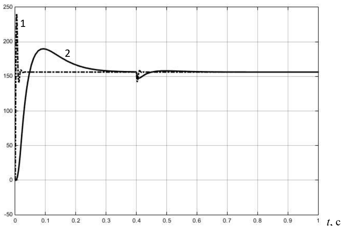
Рис. 2. Переходные характеристики контура скорости при набросе нагрузки M_c : 1 – без учета ограничения напряжения на операционном усилителе регулятора скорости; 2 – с учетом ограничения напряжения
