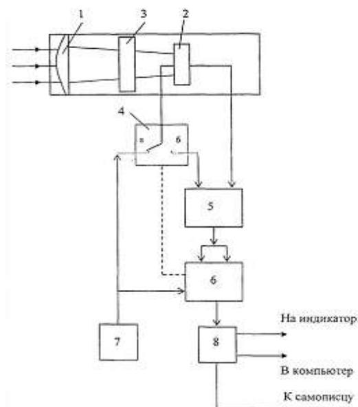
Функциональная схема пирометра спектрального отношения
