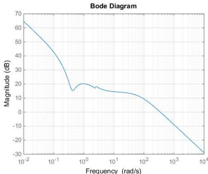
Рис. 2. Логарифмическая амплитудно-частотная характеристика корректирующего устройства
