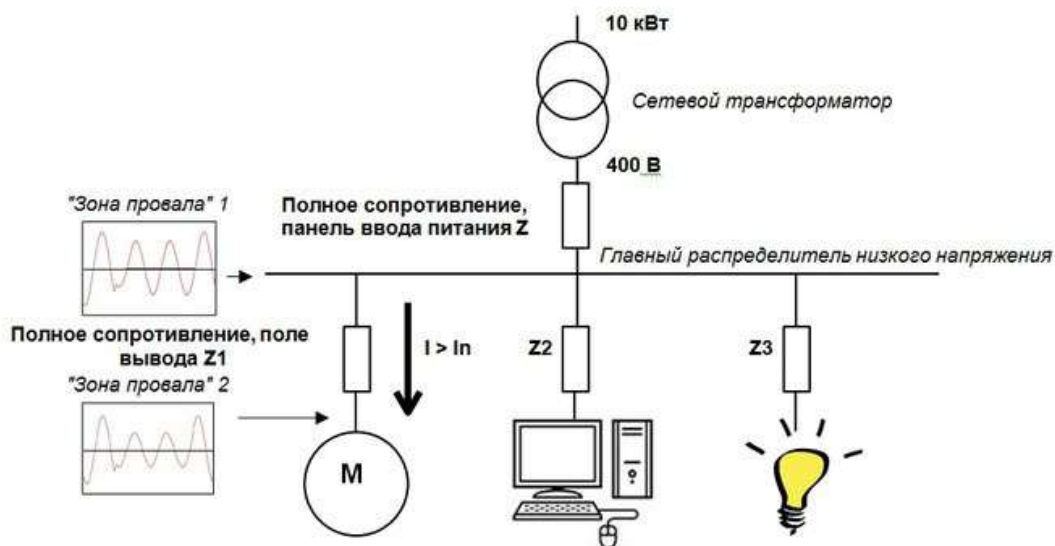
Рис. 1. «Запуск» двигателей может привести к провалу напряжения
