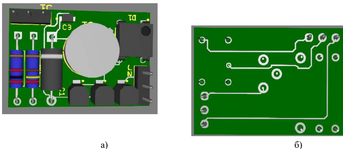
Рис. 2. 3D-модель печатной платы обработки информации в программе Ultiboard (а) вид сверху, б) вид снизу)
