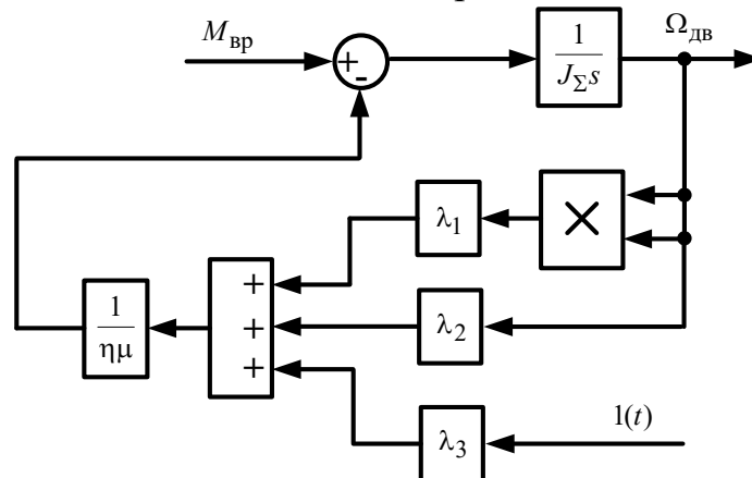
Рис. 1. Схема формирования момента сопротивления M_c(t)
