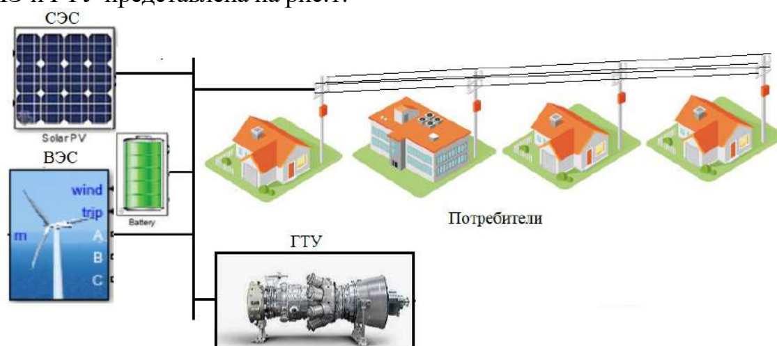
Рис.1. Принципиальная схема электроснабжения изолированного района
