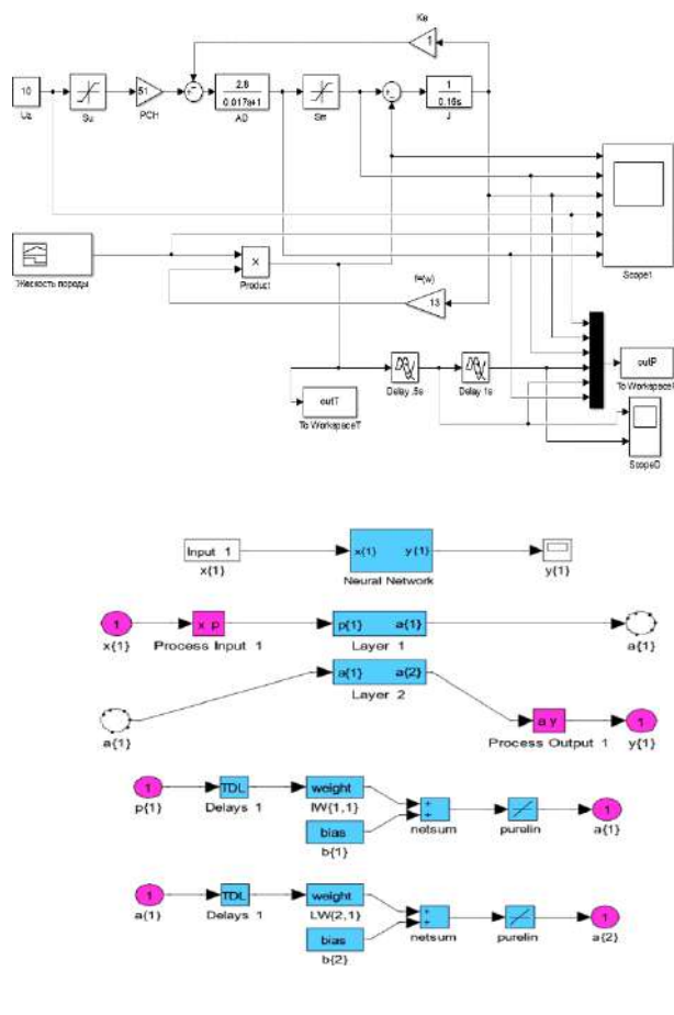
Рис.1. а) Структурная схема ЭП дробления комбайна, предназначенная для обучения нейронной сети, б) Структурная схема нейронной сети
