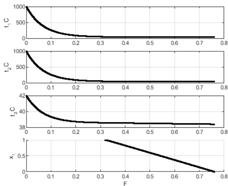
Рис. 2. Расчетные зависимости температуры ( t ) и доли водяных паров ( x ) вдоль поверхности нагрева для трех потоков теплоносителей: индекс 1 – водяные пары, 2 – сухие дымовые газы, 3 – охлаждающая вода
