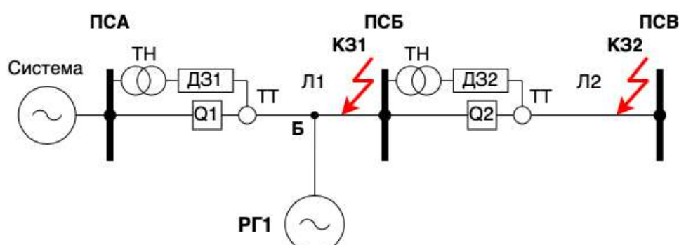
Рис. 1. Общая схема участка сети
