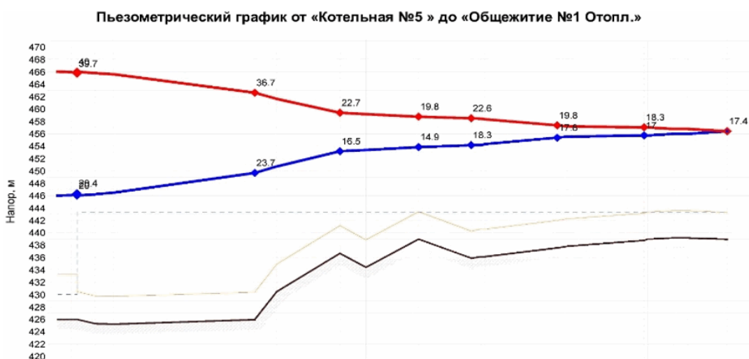
Рис. 1. Пьезометрический график до наладки
