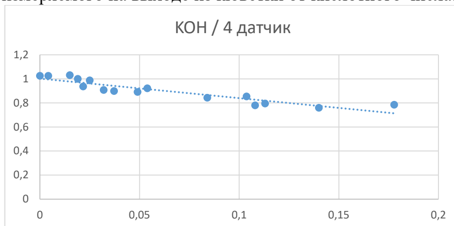
Рис 2. Зависимость кислотного числа от тока на выходе из кюветки
