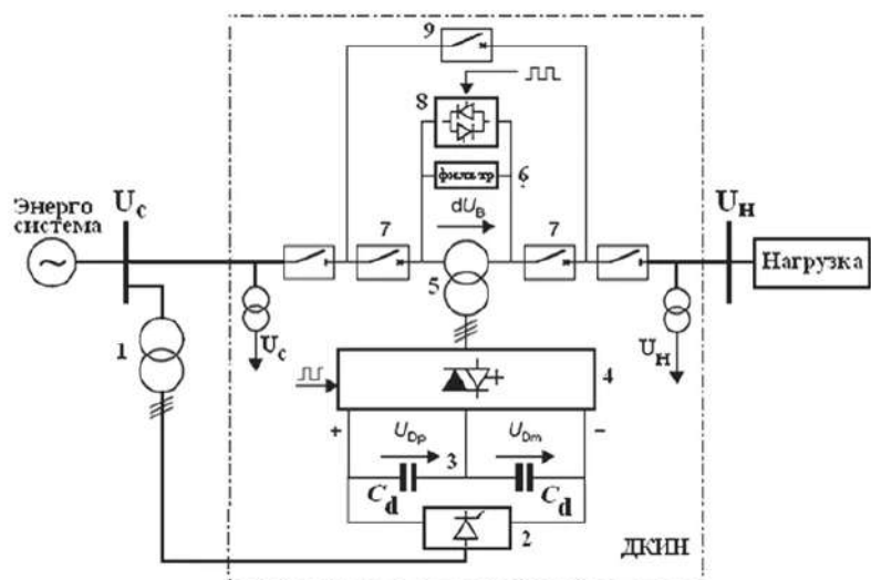
Структурная схема ДКИН
