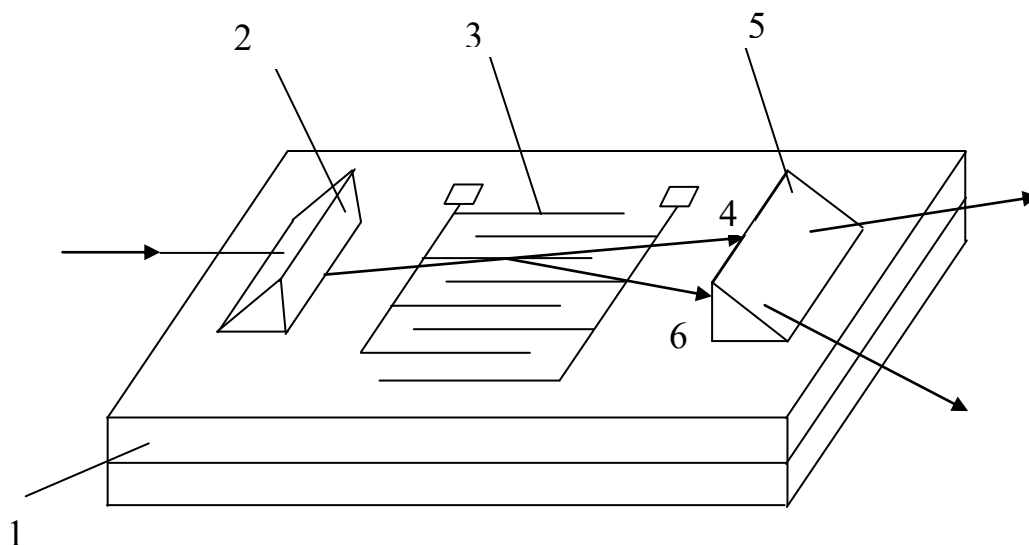
Акустооптический модулятор на поверхностных акустических волнах
