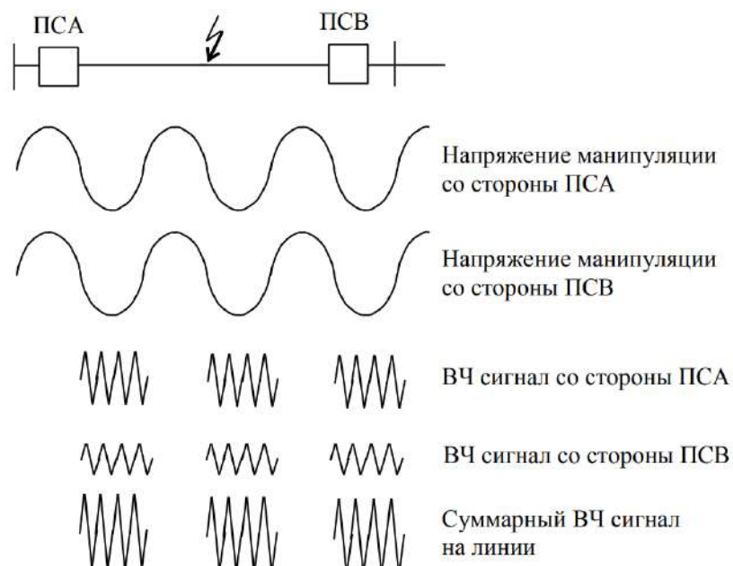
Рис. 2. Сигнала при КЗ в зоне защиты
