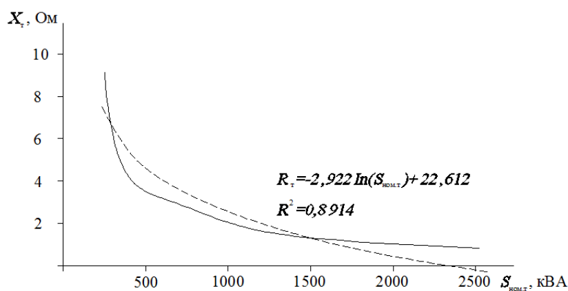
Рис. 2. Зависимость величины реактивного сопротивления X_T от номинальной мощности S_{НОМ.Т} для трансформаторов типа ТМ
