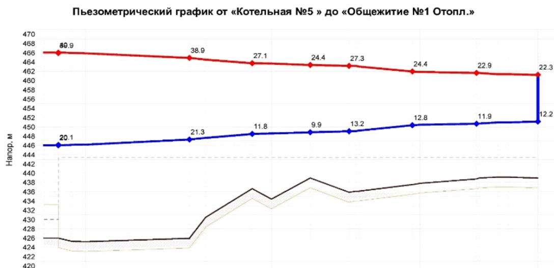
Рис. 2. Пьезометрический график после наладки
