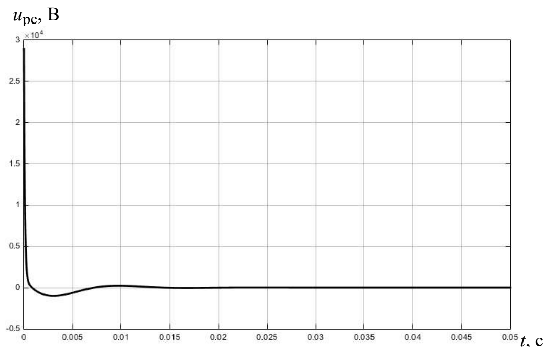
Рис.1. Напряжение на выходе регулятора скорости
