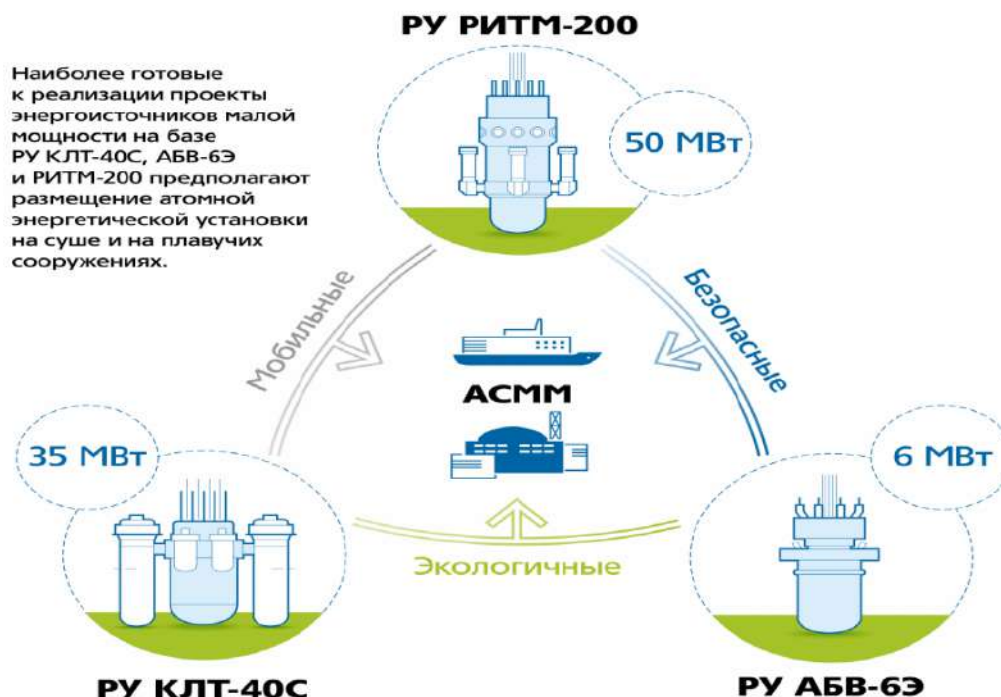
Рис. 1. АСММ на базы реактора РИТМ-200
