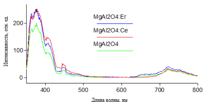
Рис. 2. Спектры люминесценции \text{MgAl}_2\text{O}_4 , \text{MgAl}_2\text{O}_4\text{:Ce} и \text{MgAl}_2\text{O}_4\text{:Er} при \lambda_{\text{ex}} = 330\text{ нм}
