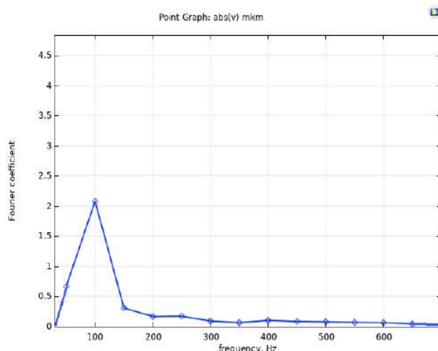
Рис. 1. Амплитудный спектр бездефектного магнитопровода
