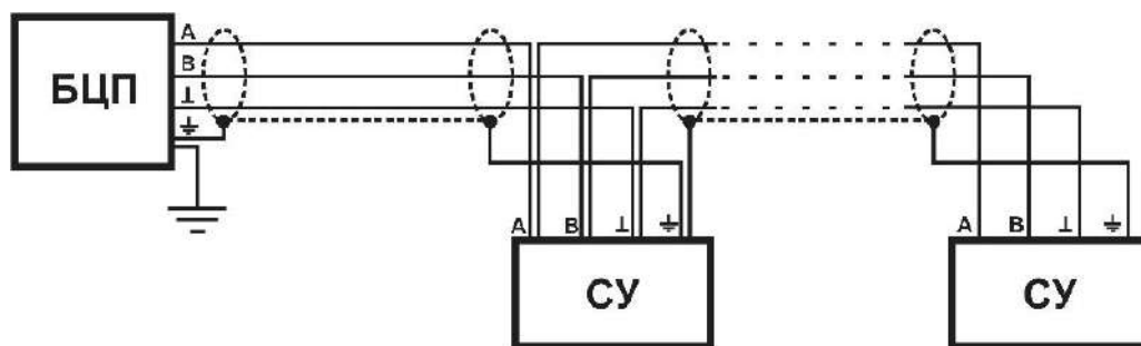
Рис. 2. Заземление БЦП
