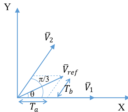
Рис. 1. График вектора опорного напряжения модуляции в секторе 1
