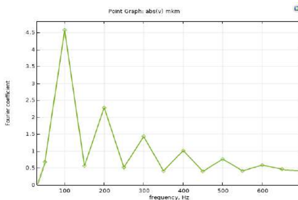
Рис. 2. Амплитудный спектр дефектного магнитопровода
