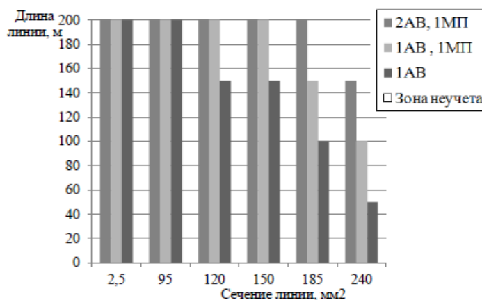
Рис.1. Зона учета сопротивлений контактной аппаратуры при определении эквивалентного сопротивления схемы с 4 кабелями
