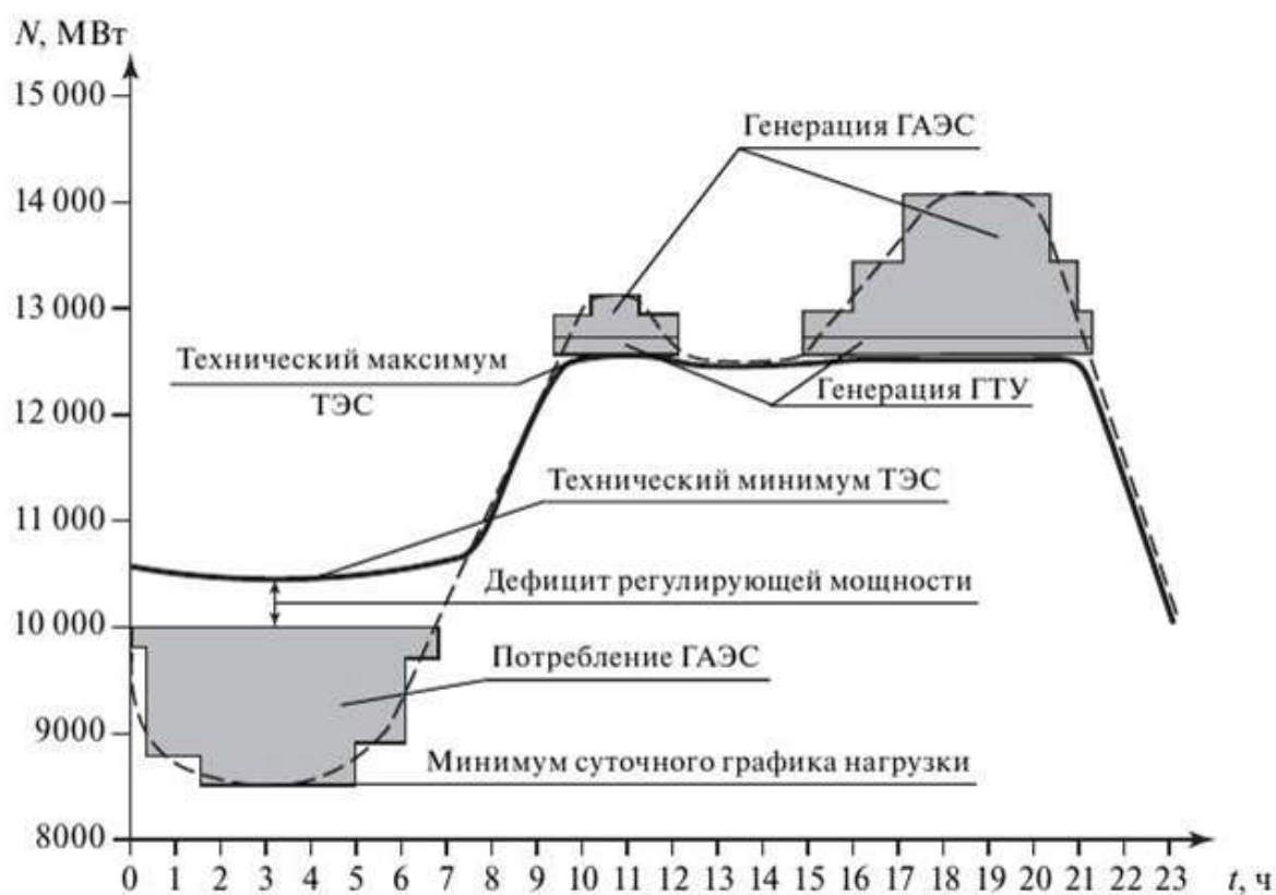
График включения гравитационной электростанции
