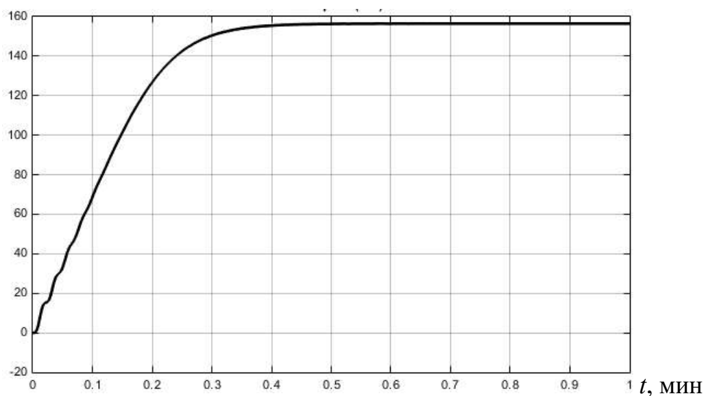
Рис. 3. Скорость движения электровоза
