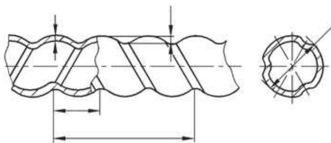
Поперечное сечение профильно-витых трубок
