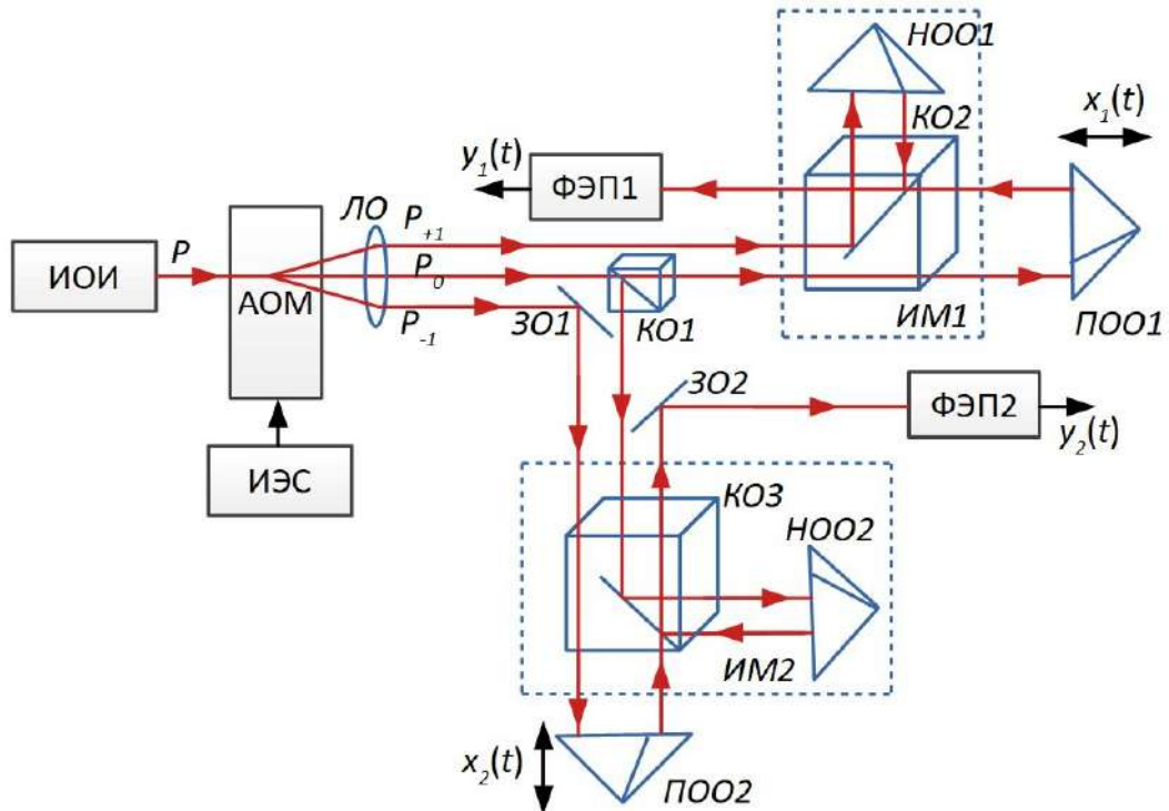
Оптическая схема информационно-измерительной системы с акустооптическим преобразованием частоты на входе интерференционной схемы.
