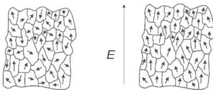
Рис. 1. Неупорядоченная поляризация и упорядоченная поляризация доменов при наложении сильного электрического поля
