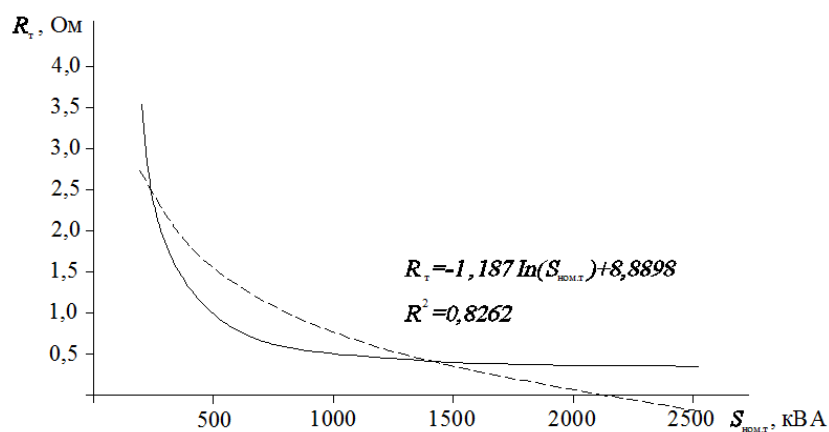
Рис. 1. Зависимость величины активного сопротивления R_T от номинальной мощности S_{НОМ.Т} для трансформаторов типа ТМ
