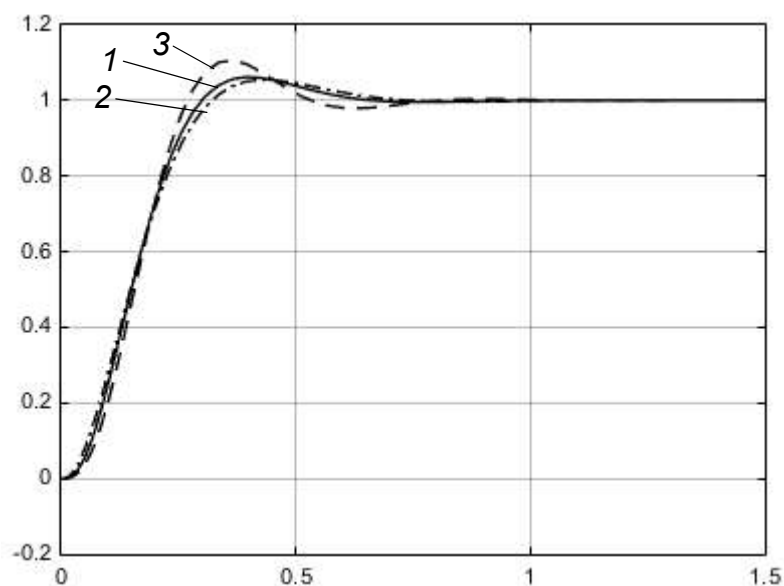
Рис. 2. Переходные характеристики электромеханической системы с компенсационным алгоритмом управления: 1) a_1 = 4; a_0 = 2; b_0 = 5 ; 2) a_1 = 8; a_0 = 4; b_0 = 10 ; 3) a_1 = 2; a_0 = 1; b_0 = 2,5
