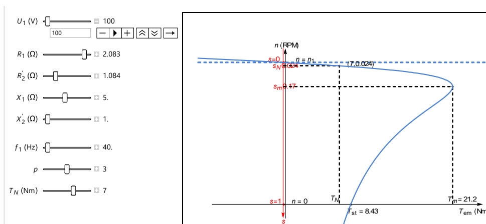
Рис. 1. Панель моделирования статической характеристики АД – зависимости частоты вращения от электромагнитного момента при изменении напряжения статора. а) U_1=200 В, б) U_1=150 В, в) U_1=100 В
