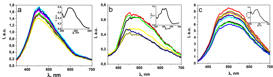
Рис.3 Спектры ФЛ образцов
