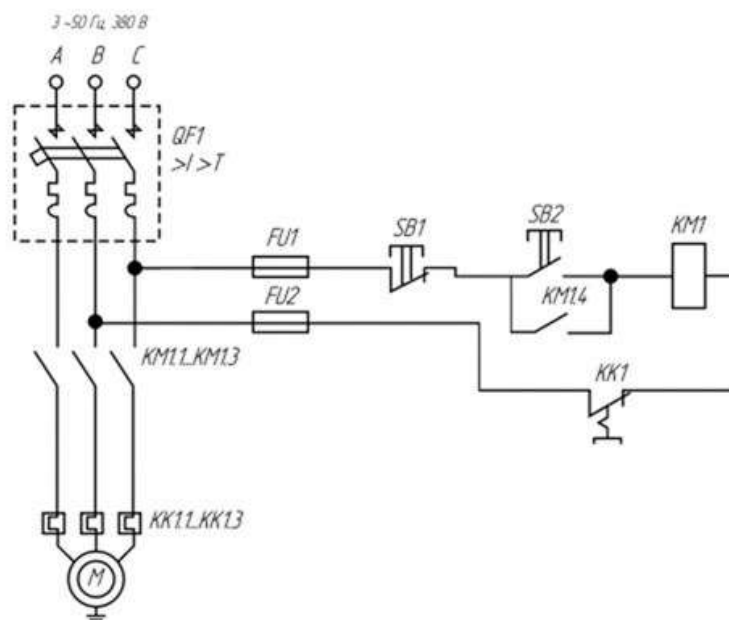
Рис. 2. Электрическая схема электропривода насоса до модернизации
