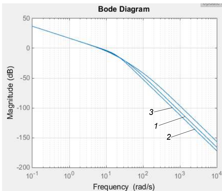
Рис. 3. Логарифмические амплитудно-частотные характеристики электромеханической системы с компенсационным алгоритмом управления: 1) a_1 = 4; a_0 = 2; b_0 = 5 ; 2) a_1 = 8; a_0 = 4; b_0 = 10 ; 3) a_1 = 2; a_0 = 1; b_0 = 2,5
