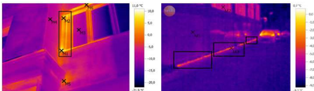
Рис. 3. Пример локального выявления тепловых потерь при энергетическом (тепловизионном) обследовании многоквартирного жилого дома в городе Вологде
