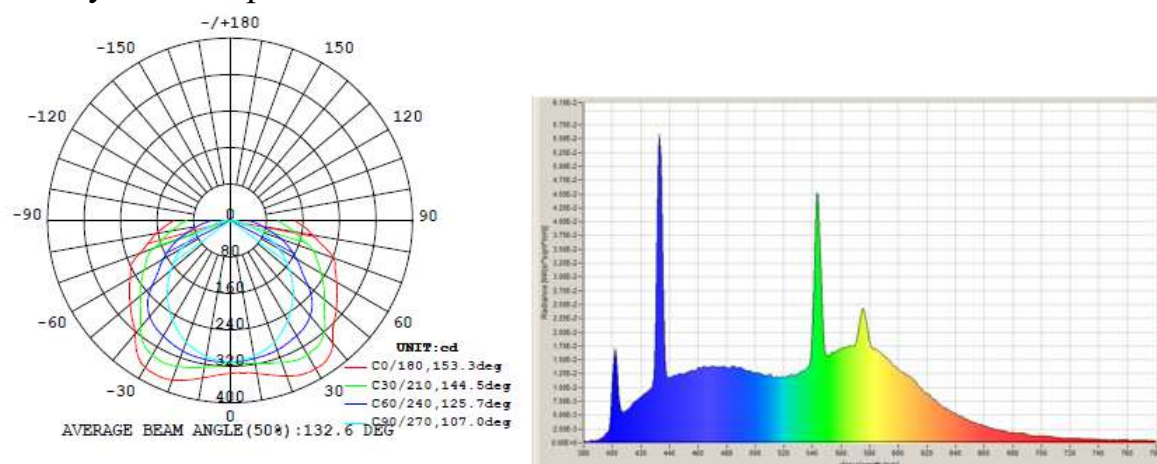
Рис. 1. КСС и спектр исследуемого образца светильника
