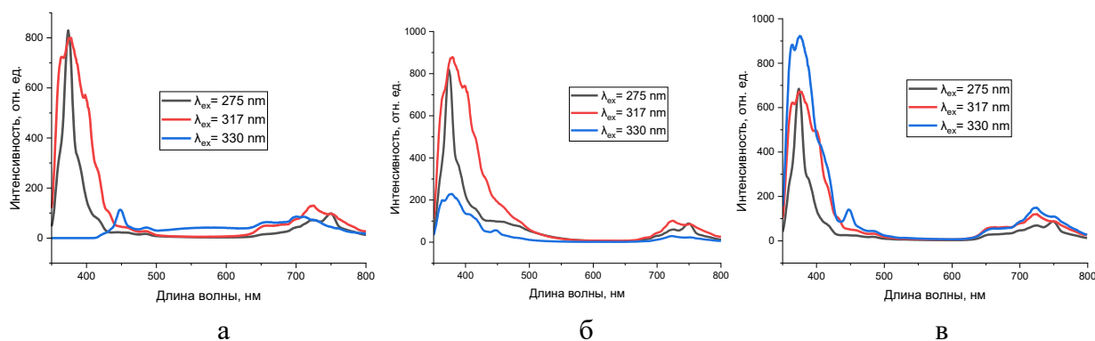
Рис. 1. Спектр ФЛ \text{MgAl}_2\text{O}_4 (а), \text{MgAl}_2\text{O}_4:\text{Ce}^{3+} (б) и \text{MgAl}_2\text{O}_4:\text{Er}^{3+} (в)
