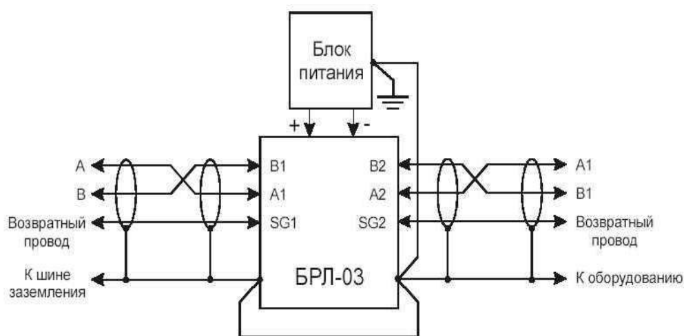
Рис. 1. Схема подключения БРЛ в линию связи
