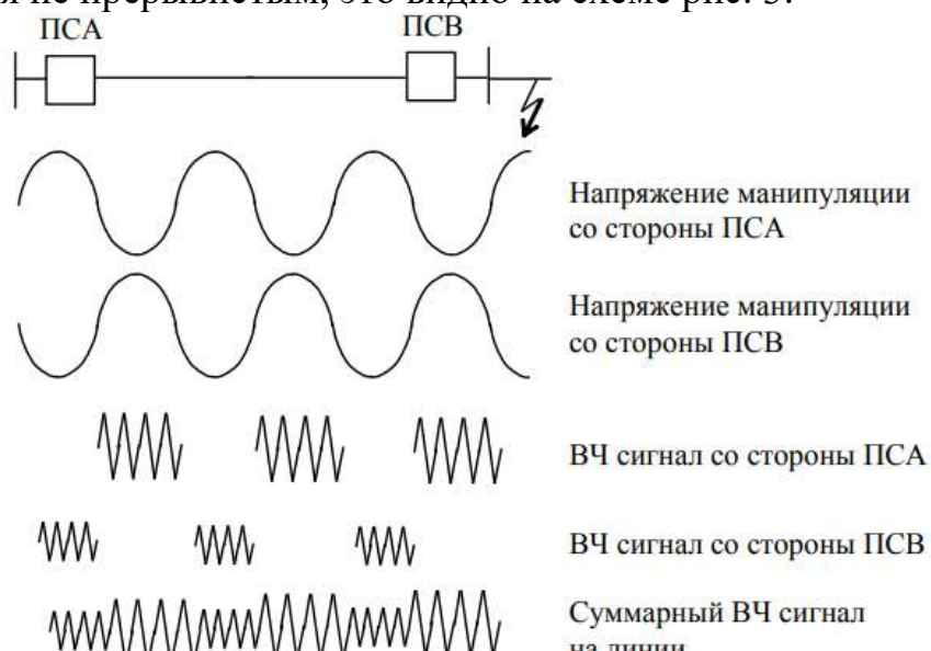
Рис. 3. Сигнала при КЗ в зоне защиты
