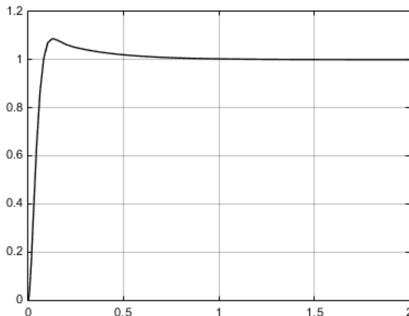
Рис. 3. График переходного процесса скорректированной анемометрической системы
