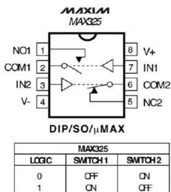
Рис. 2 Распиновка аналогового ключа
