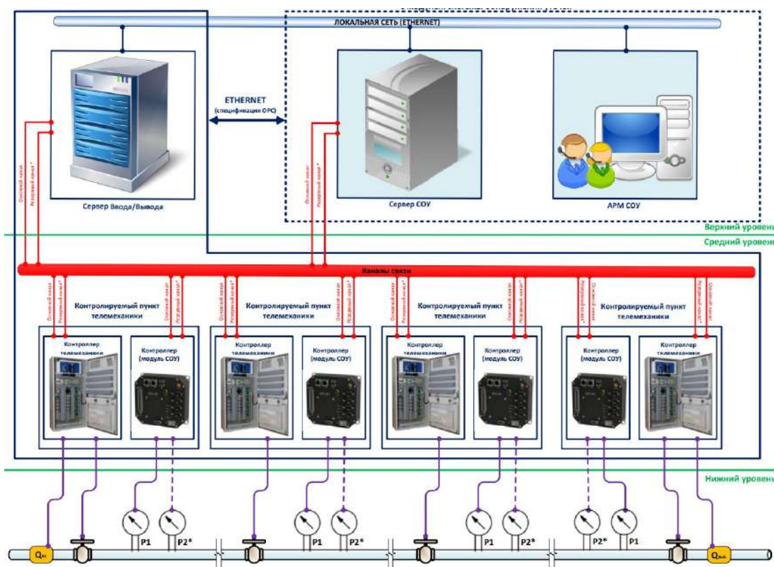
Структурная схема ПТК СОУ
