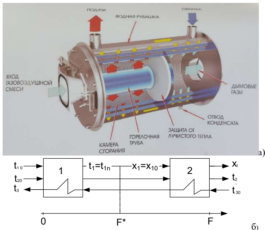
Рис. 1. Продольный разрез котла GEFFEN MB с указанием направления потоков теплоносителей (а) и его расчетная схема (б)
