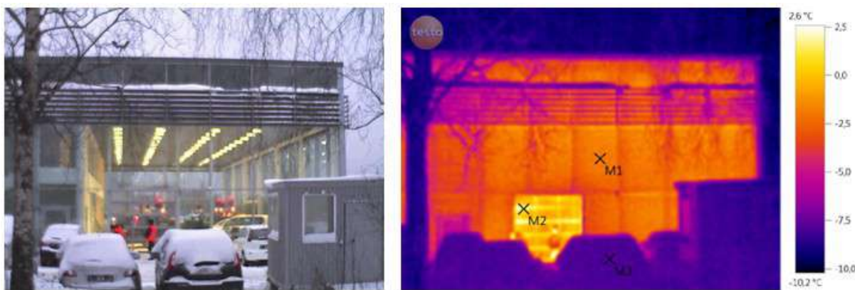
Рис. 4. Пример визуального цифрового (слева) и теплового (справа) контроля наружных ограждающих конструкций торгово-сервисного центра в городе Вологде
