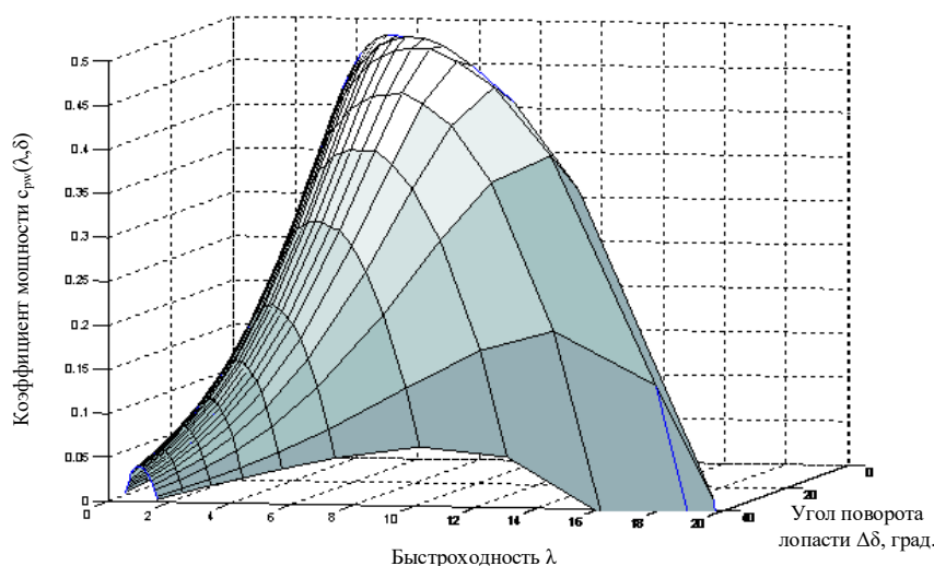
Рис. 1. Расчетная зависимость коэффициента мощности ветроколеса c_{pw} от быстроходности \lambda и углом поворота лопасти \Delta\delta [2]
