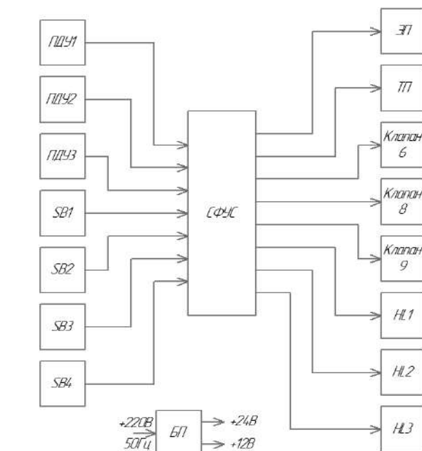
Структурно-функциональная схема информационно-измерительного канала управления мобильной снегоплавильной установки
