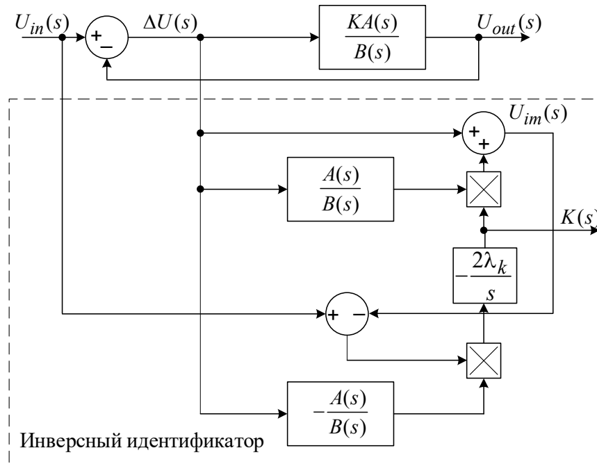
Структурная схема динамической модели идентификации статического коэффициента передачи электропривода
