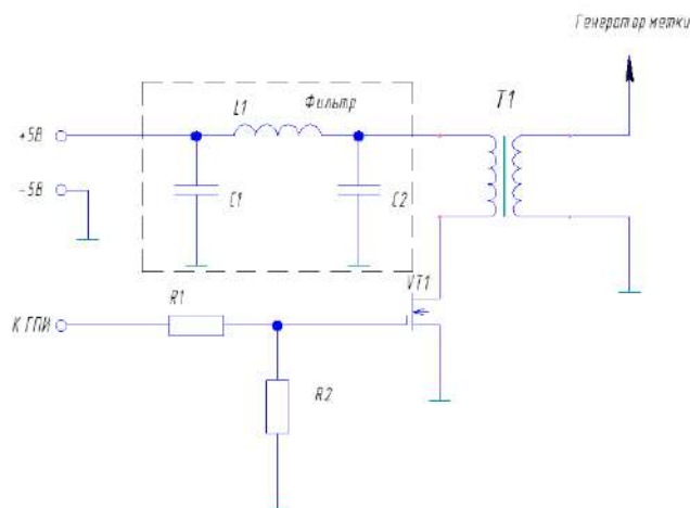
Рис.1 Генератор высоковольтных импульсов
