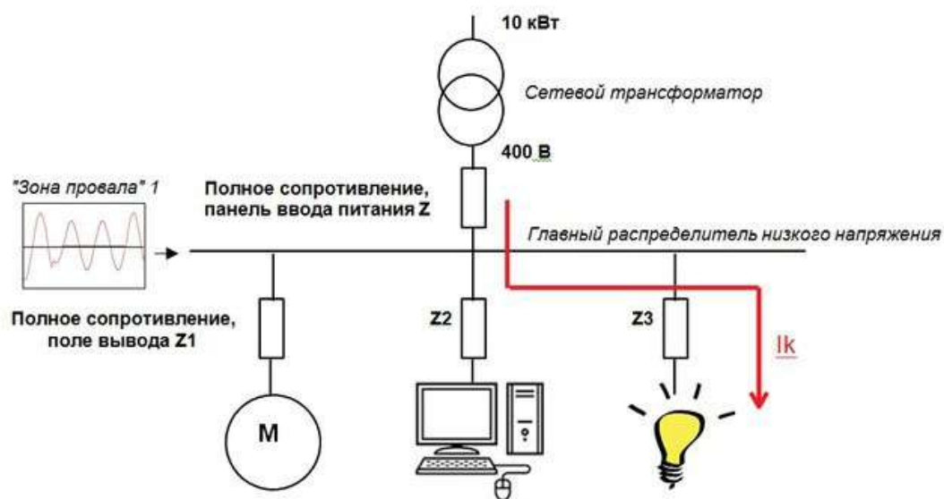
Рис. 2 Типичный пример рабочего состояния, при котором провал напряжения возникает в результате короткого замыкания в сети низкого напряжения
