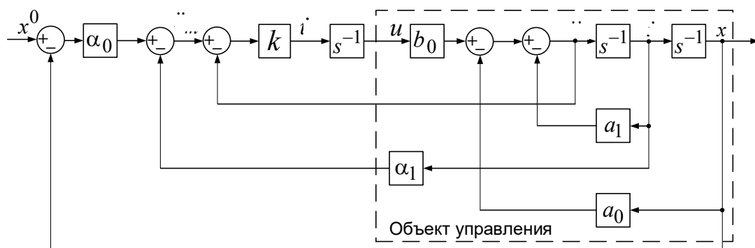
Рис. 1. Структурная схема электромеханической системы с эталонной моделью
