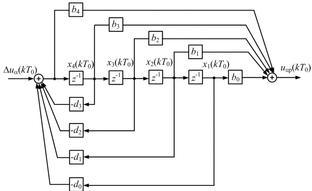
Рис. 2. Структурная схема непосредственного программирования цифрового фильтра
