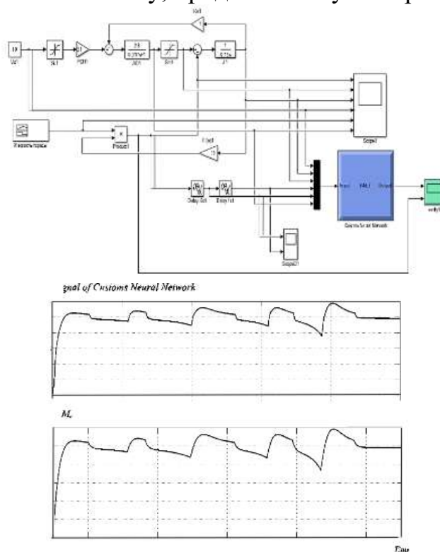
Рис. 4. а) Структурная схема ЭП дробления угольного комбайна с нейронной сетью, б) Графики идентификации момента сопротивления нейронной сетью и момента сопротивления M_c
