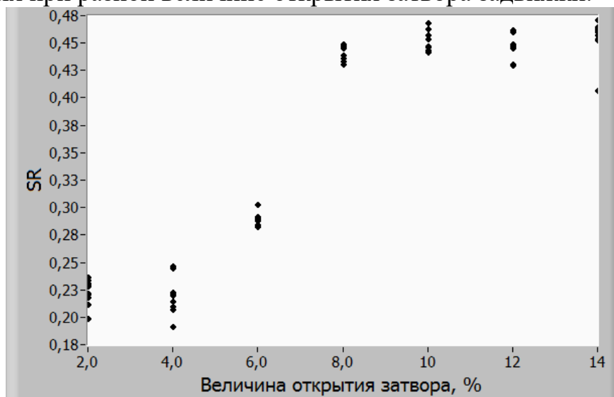
Рис. 2. Изменение параметра SR от величины открытия затвора задвижки
