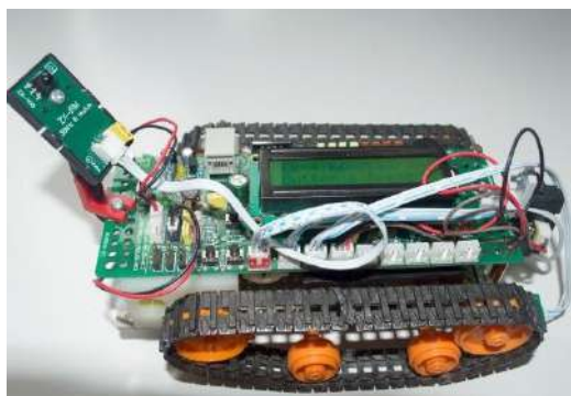
Рис. 1. Робототехническая платформа ROBOPICA
