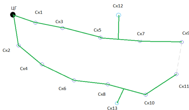
Рис. 2. конфигурация системы электроснабжения в пустынном и степном районе с дополнительными скважинами
