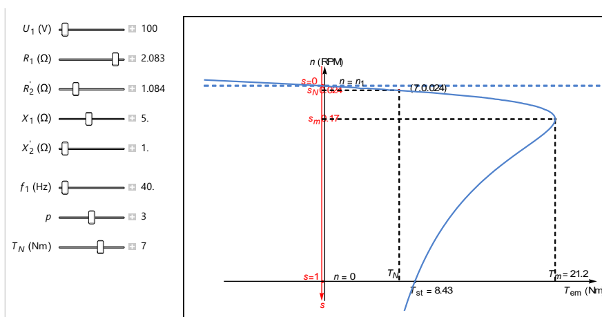
Рис. 1. Панель моделирования статической характеристики АД – зависимости частоты вращения от электромагнитного момента при изменении напряжения статора. а) U_1=200 В, б) U_1=150 В, в) U_1=100 В
