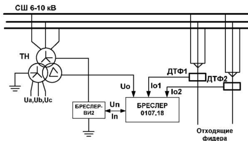
Схема подключения элементов комплекса
