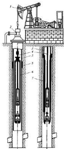
Штанговая насосная установка
