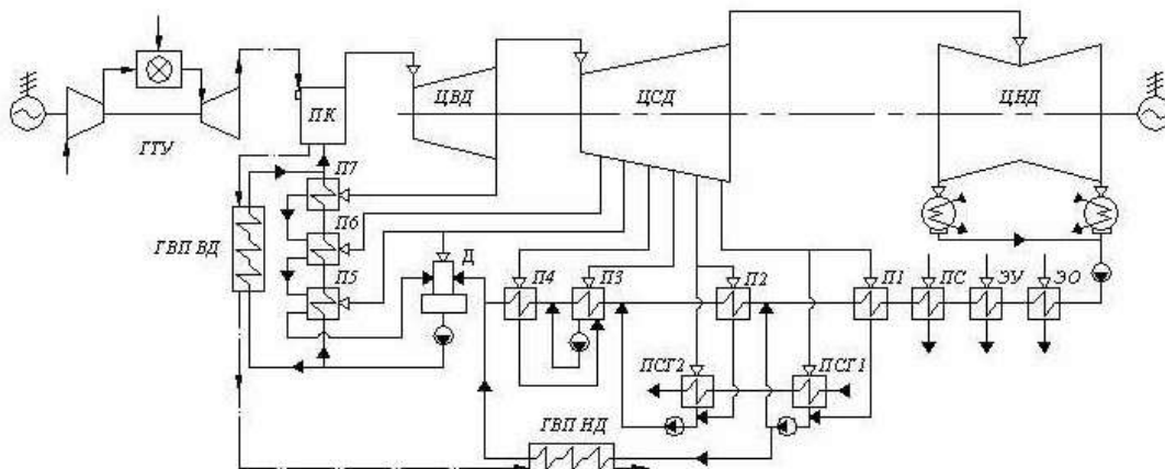
Рис. 1. Принципиальная тепловая схема ПГУ НПГ (со сбросом в ПК) с паровой турбиной Т-100/120-130. ГТУ – газотурбинная установка; ПК – паровой котел; ГВП – газ-водяной подогреватель; ПСГ – подогреватель сетевой воды горизонтального типа; Д – деаэратор; ЭУ – эжектор уплотнений; ЭО – эжектор основной; ПС – подогреватель сальниковый.
