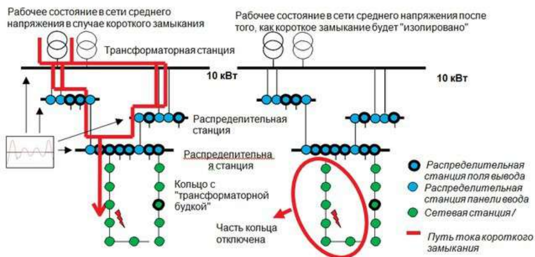
Рис. 3 Типичная структура сети среднего напряжения
