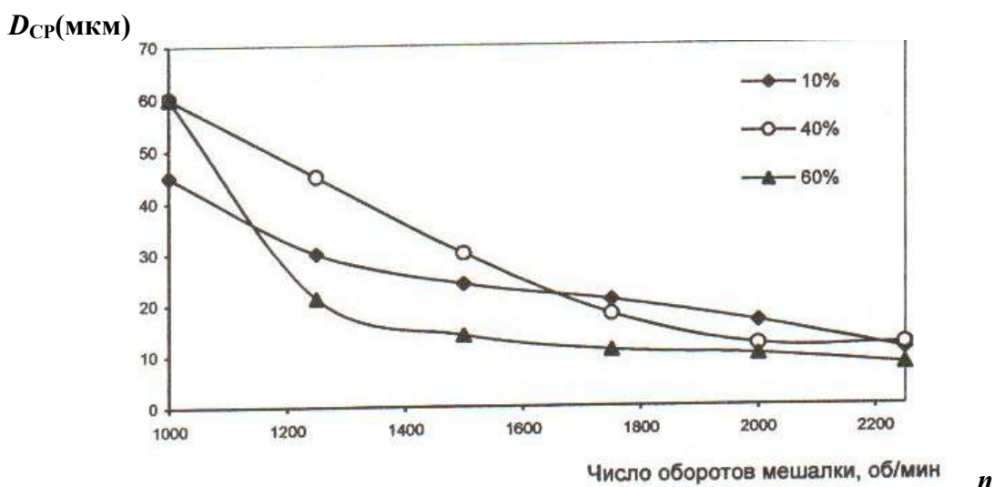
Рис.1. Зависимость среднеарифметического диаметра D_{cp} капле эмульсий нефти разной обводненности (10, 40, 60%) от числа оборотов n мешалки
