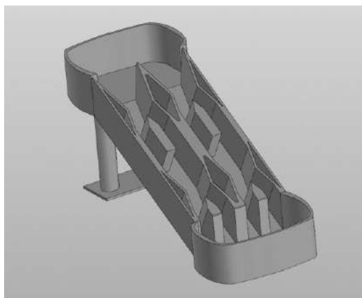
Рис. 4. 3D-модель упрощенной конструкции ГЭУ
