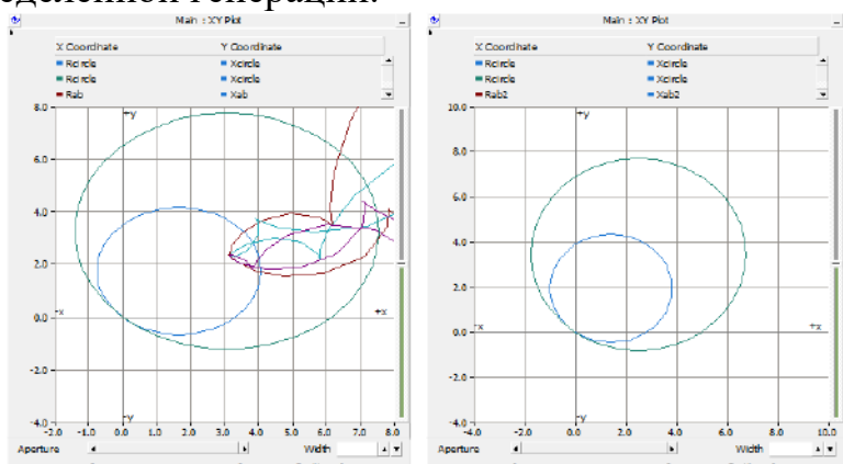
Рис. 4. Характеристики срабатывания реле сопротивления дистанционной защиты, уставки с учетом РГ (слева – Д31, справа – Д32)
