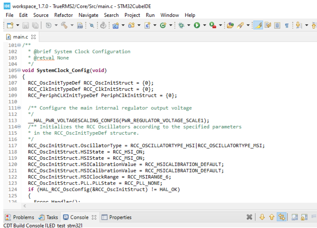
Рис. 4 Фрагмент программного обеспечения микроконтроллера
