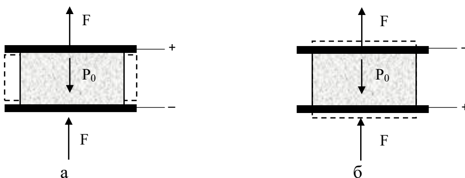
Рис. 2. Продольная деформация растяжения и сжатия пьезоэлемента
