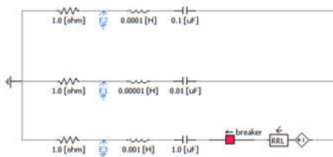
Двухконтурная схема
