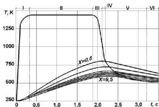
Рис. 2. Зависимость температуры основного потока ( T_0 ), обтекаемой поверхности ( T_w ) от времени и продольной координаты X
