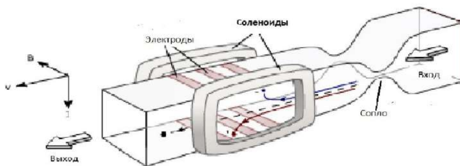
Устройство МГД-генератора
