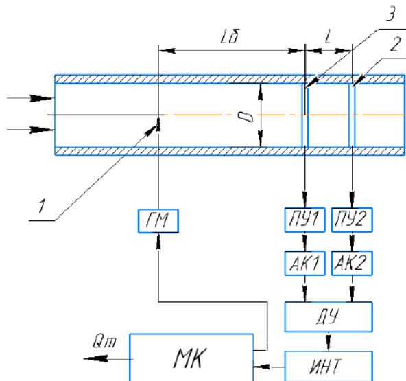
Структурно-функциональная схема ИМИРВ
