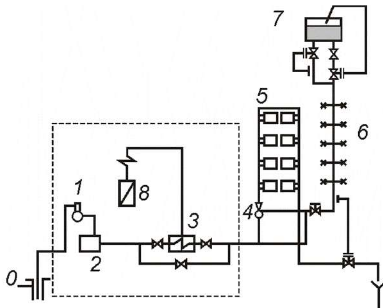
Рис. 2. 1 – дегазатор; 2 – химводоочистка; 3 – водоподогреватель; 4 – смеситель; 5 – система отопления; 6 – система горячего водоснабжения; 7 – бак-аккумулятор; 8 – котельная
