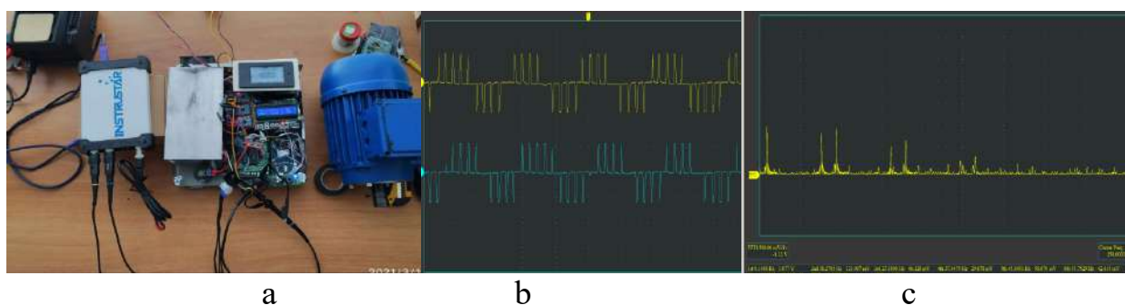
Рис 2. Модель инвертора SVPWM (а), формы волны (b) и гармоники (с).
