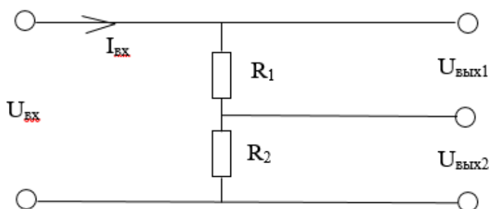
Рис. 1. Общий вид схемы делителя напряжения на резисторах
