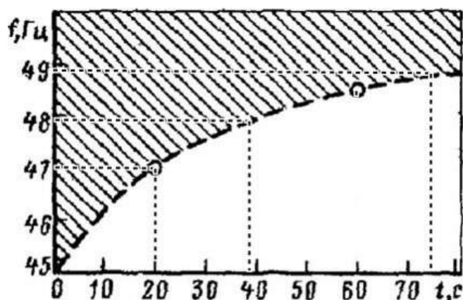
Рис. 2. Частотно-временная характеристика
