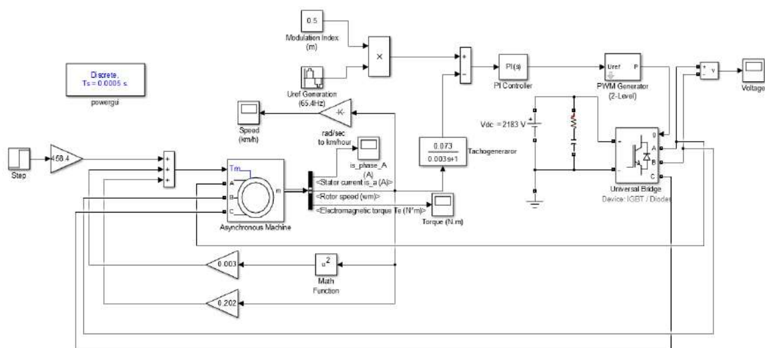
Рис. 2. Simulink -модель системы управления асинхронного тягового электропривода с автономным инвертором напряжения
