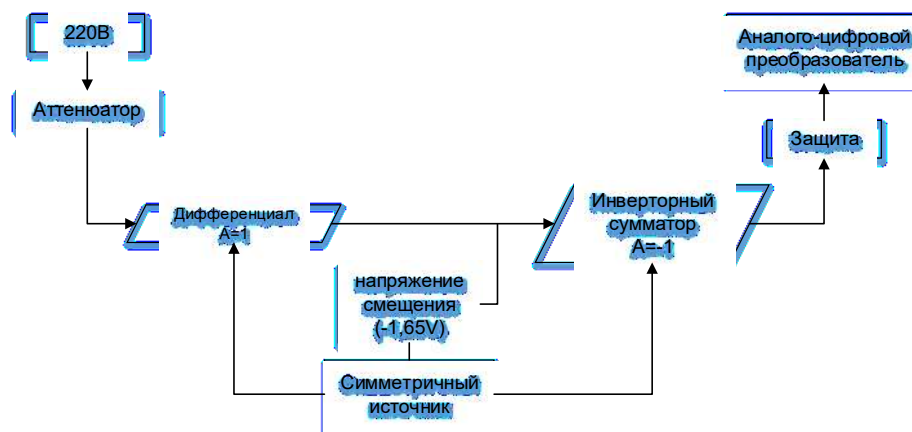
Рис 1 Блок схема измерителя TrueRMS значений
