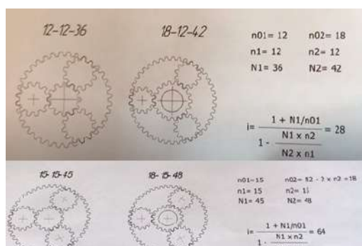
Рис.1. Схема планетарных редукторов для робота
