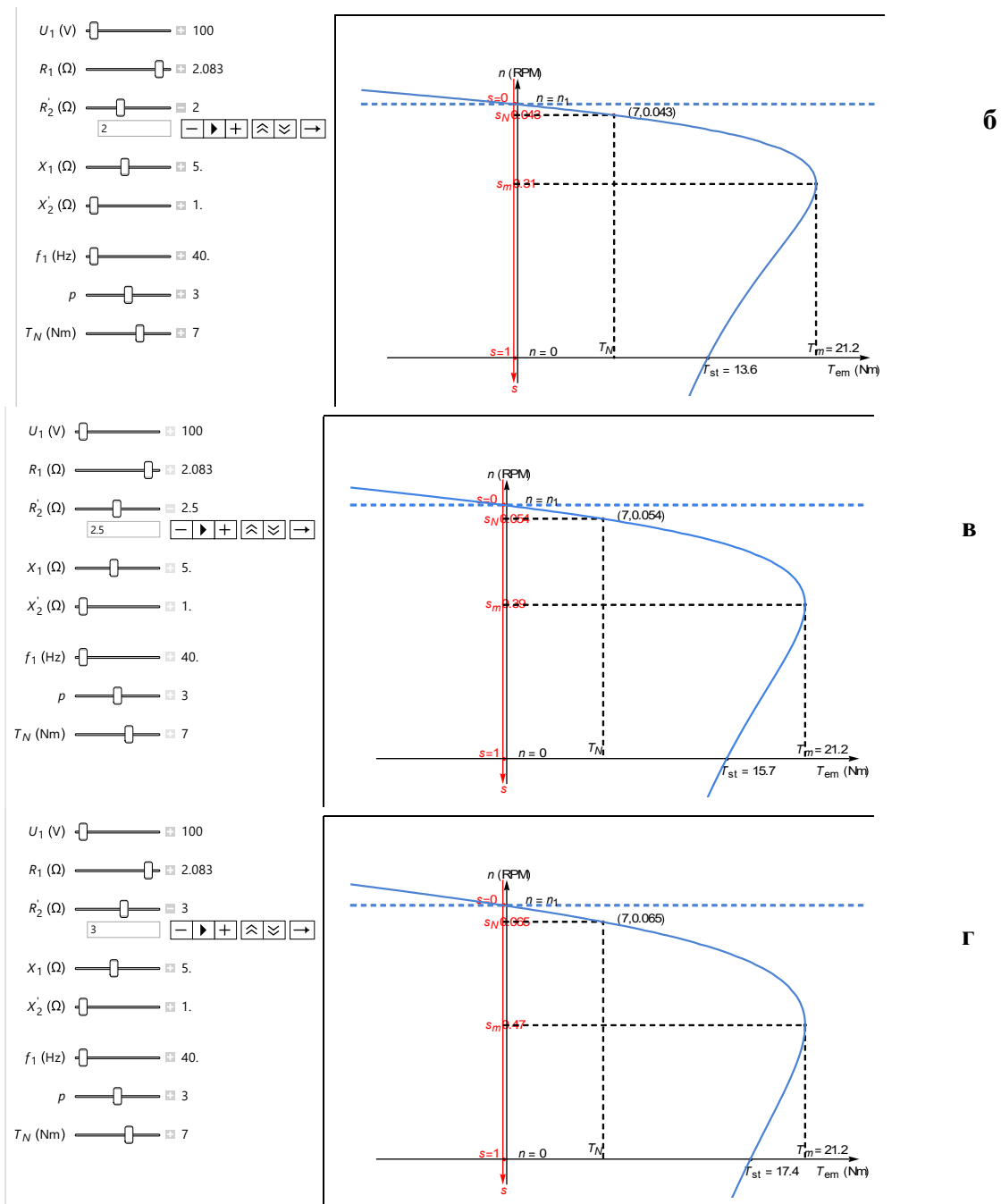
Рис. 2. Панель моделирования статической характеристики при изменении добавочного сопротивления ротора. а) R_2' = 1 Ом, б) 2 Ом, в) 2,5 Ом, г) 3 Ом
