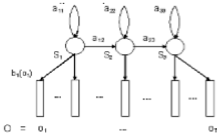
Рис. 2. СММ с тремя состояниями
