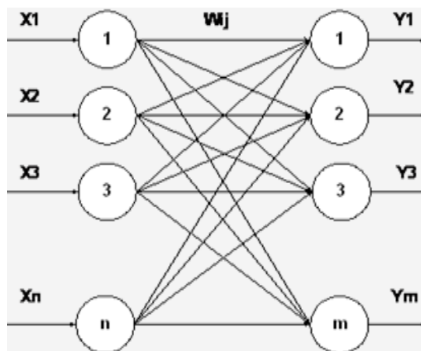
Рис. 3. Пример однослойной нейронной сети
