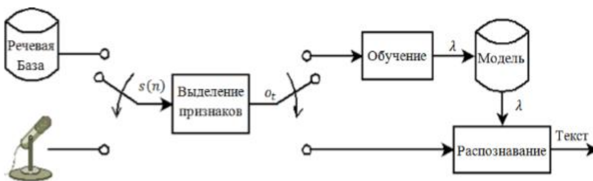
Рис. 1. Общая схема системы автоматического распознавания речи
