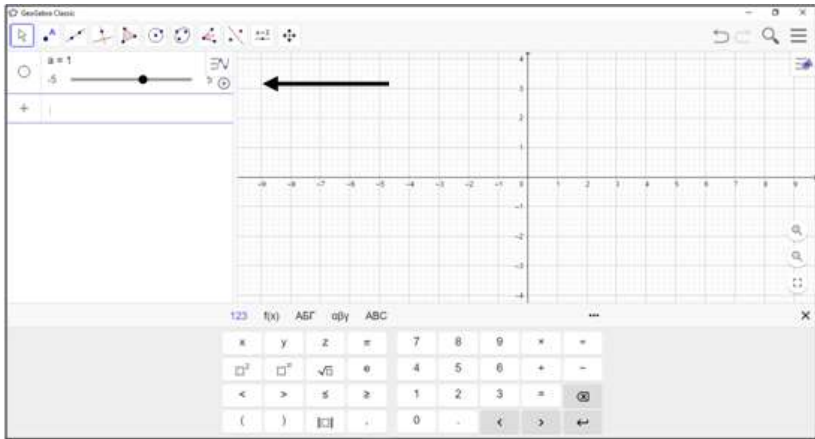
Рисунок 2 – Создание ползунка для коэффициента a
