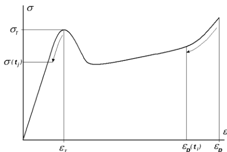
Рис. 2. Схема кинетики изменения диаграммы деформирования ( \sigma - \epsilon ) образцов свидетелей, вырезанных из полиэтиленового трубопровода в процессе мониторинга.
