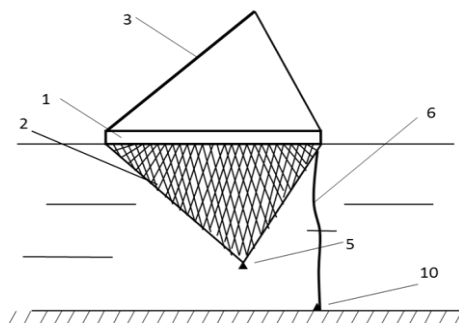
Рисунок 4. Рабочее положение устройства и ставной сети, вид сбоку
