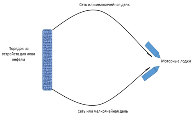
Рисунок 8. Способ обхвата мелких нагульных групп кефали и направление её движения к отлавливающему устройству
