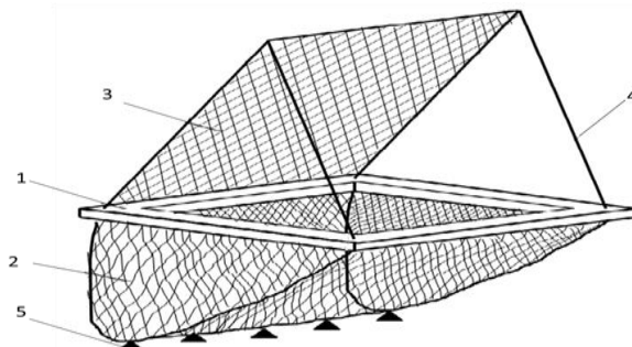
Рисунок 2. Общий вид устройства
