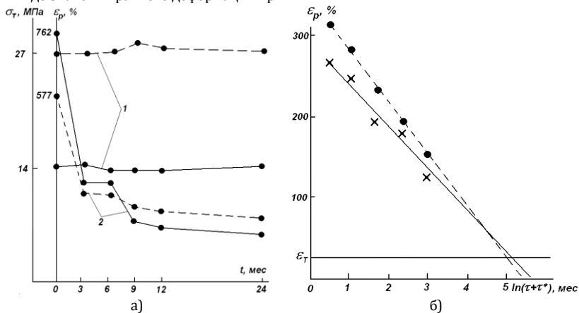
Рис. 1. а) зависимость \sigma_t (1) и \epsilon_p (2) полиэтиленов от времени теплового старения; б) определение предельного срока службы полиэтиленов: ПЭНП (-) и ПЭВП (---)
