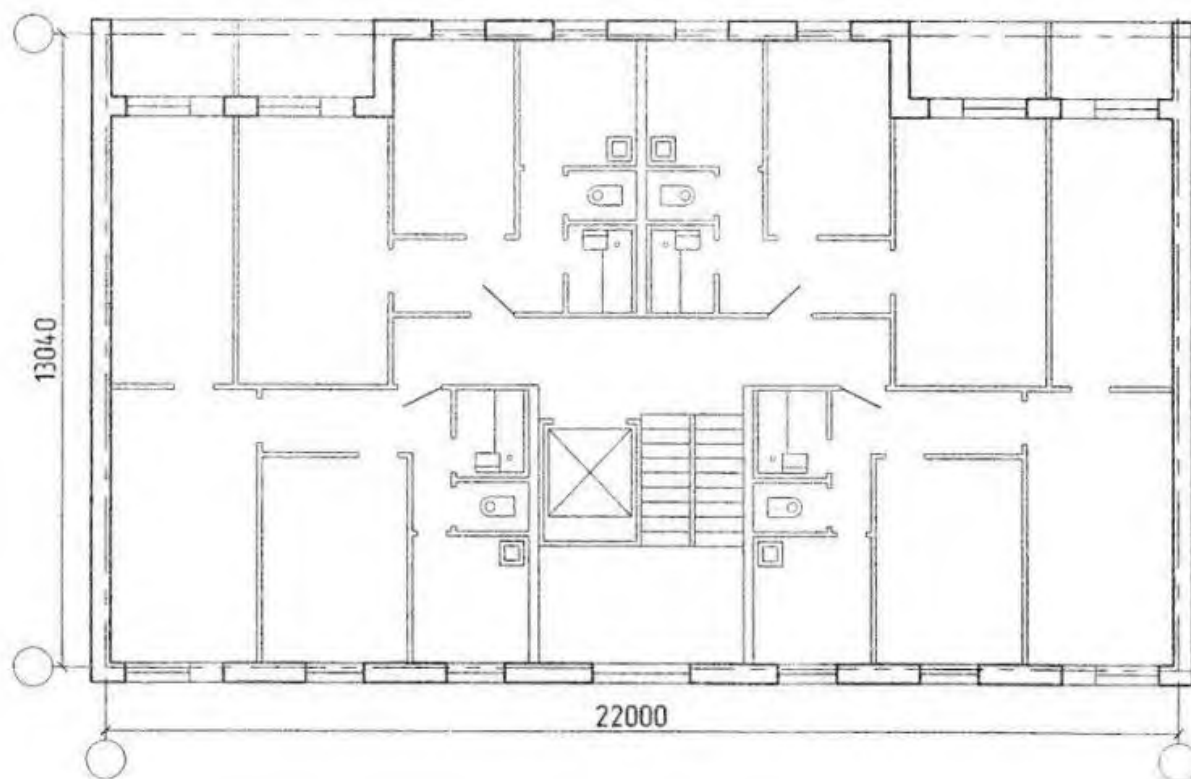
План типовой секции жилого дома серии 464 (масштаб 1:100)
