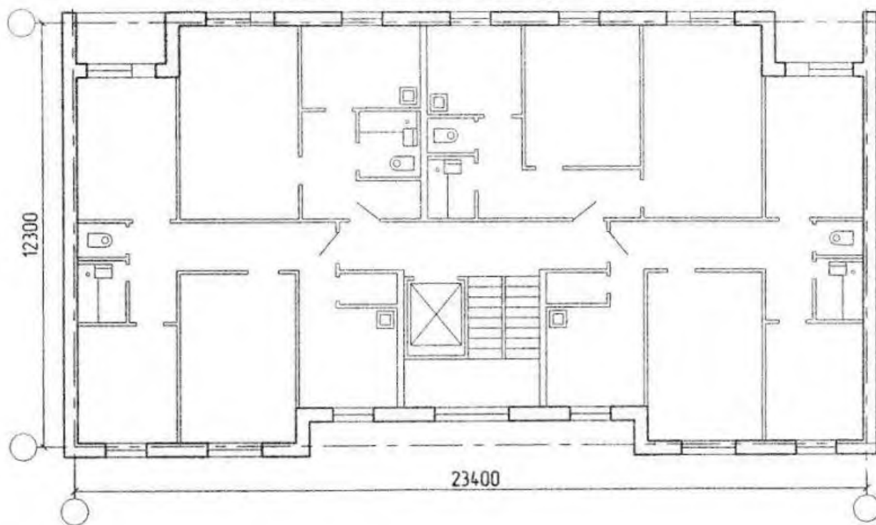
План типовой секции жилого дома серии 90 (масштаб 1:100)
