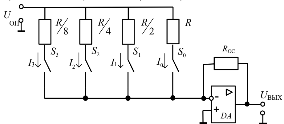
Рис. 10. Схема ЦАП с двоично-взвешенными резисторами
