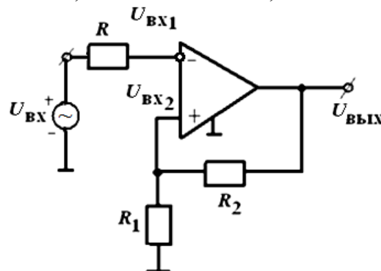
Рис. 7. Триггер Шмитта на ОУ
