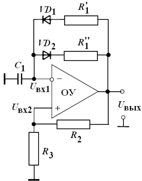
Рис. 8. Несимметричный мультивибратор на ОУ
