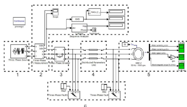
Рисунок 1. Модель электрической сети с изолированной нейтралью
