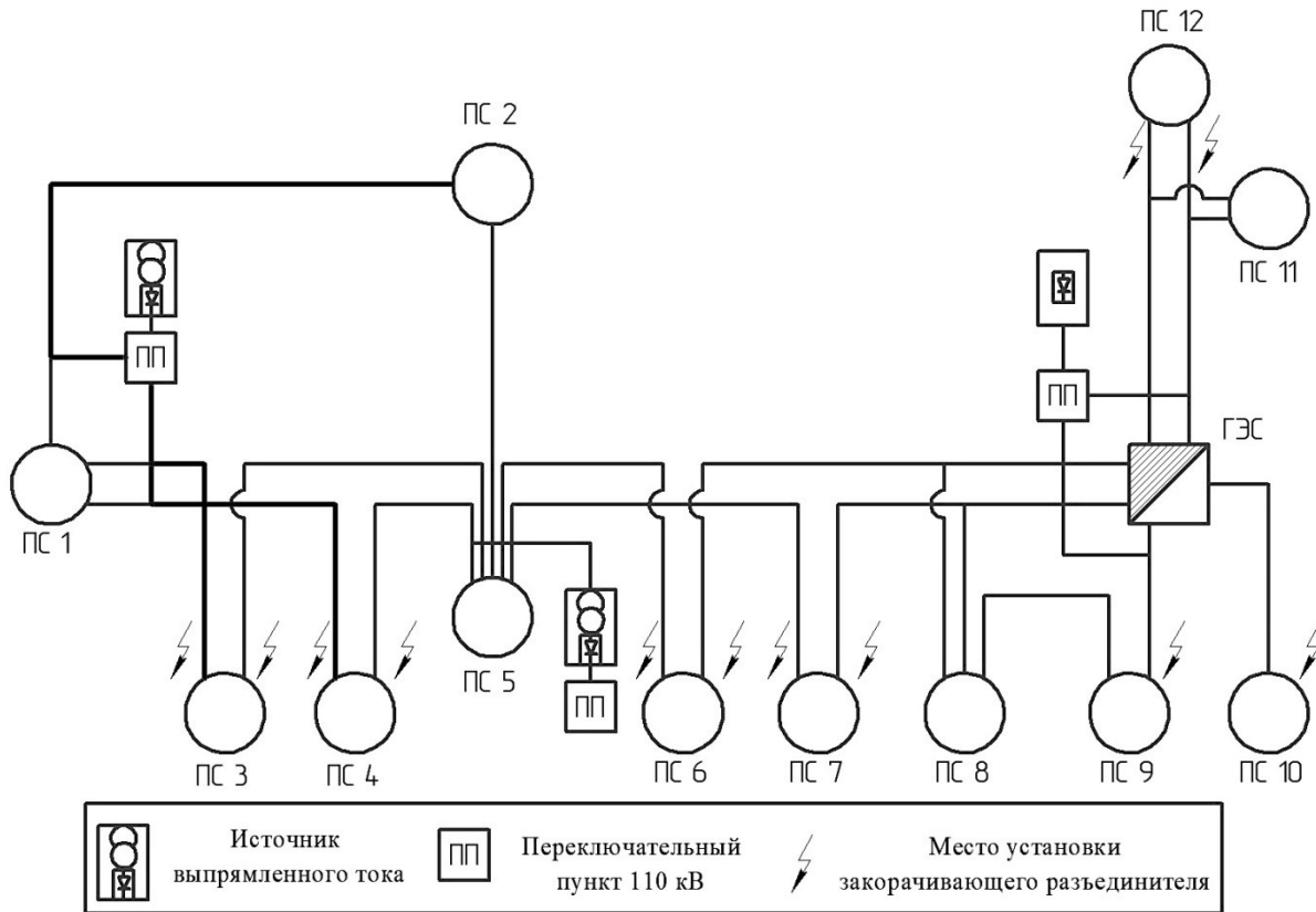
Рисунок 1. Схема плавки гололеда постоянным током
