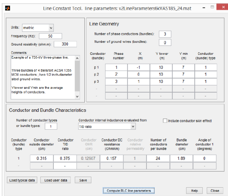
Рисунок 2. Окно расчёта параметров линии электропередач
