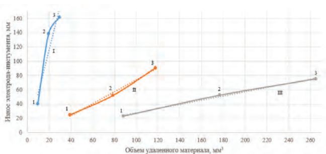
Рисунок 1. Зависимость износа электрода - инструмента от объема удаленного материала, I – диаметр электрода 0,5 мм; II - диаметр электрода 1,0 мм; III - диаметр электрода 1,5 мм; 1 – глубина обработки 50 мм, 2 – глубина обработки 100 мм, 3 – глубина обработки 150 мм
