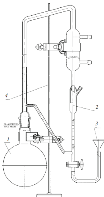
Рисунок 1. Установка для отгонки эфирных масел: 1 – испарительная колба, 2 – система охлаждения, 3 – воронка лабораторная, 4 – штатив
