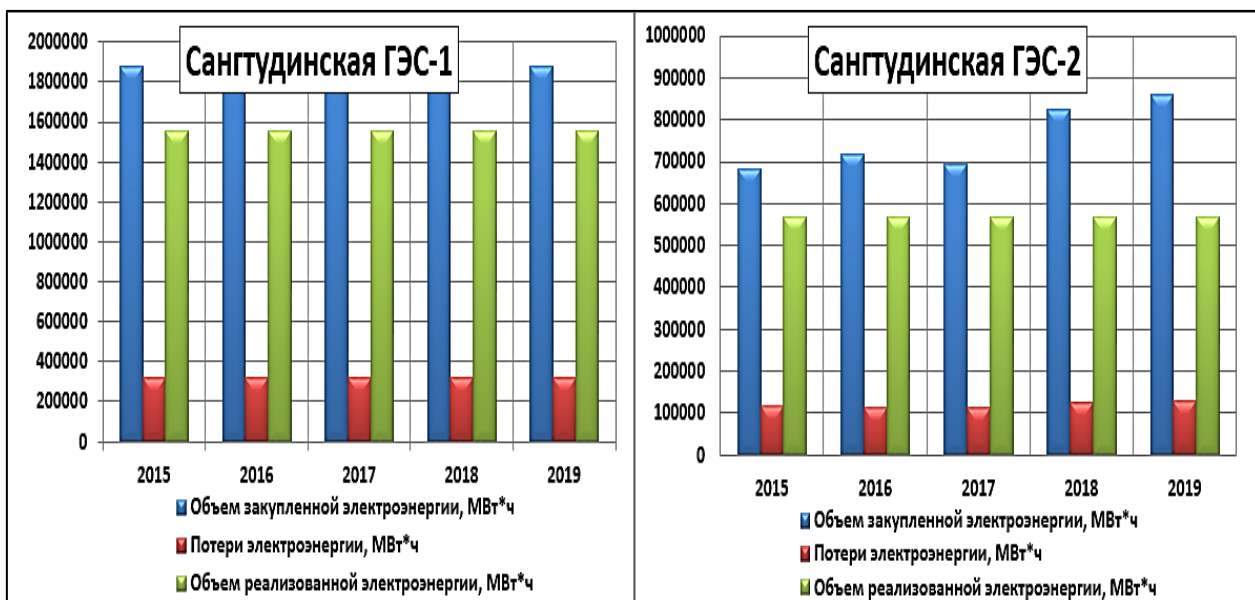
Рисунок 86. Объемы закупки, реализации и потерь электроэнергии, мВт.час в 2015-2019 гг.
