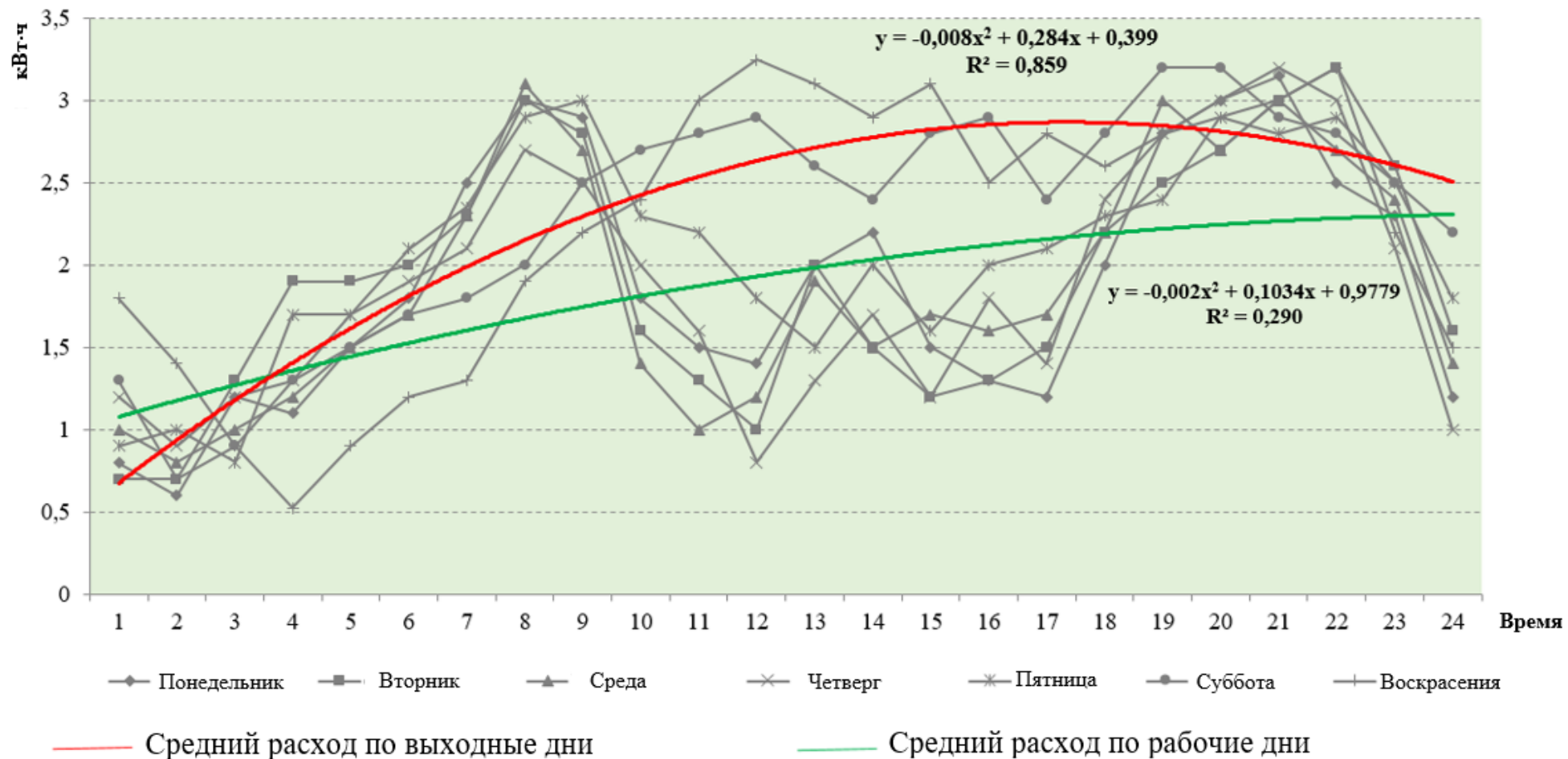
Рисунок 157. Графики почасового изменения потребления электрической энергии в мае 2019 года населением Бектемирского района (месяц минимального потребления электрической энергии в году)
