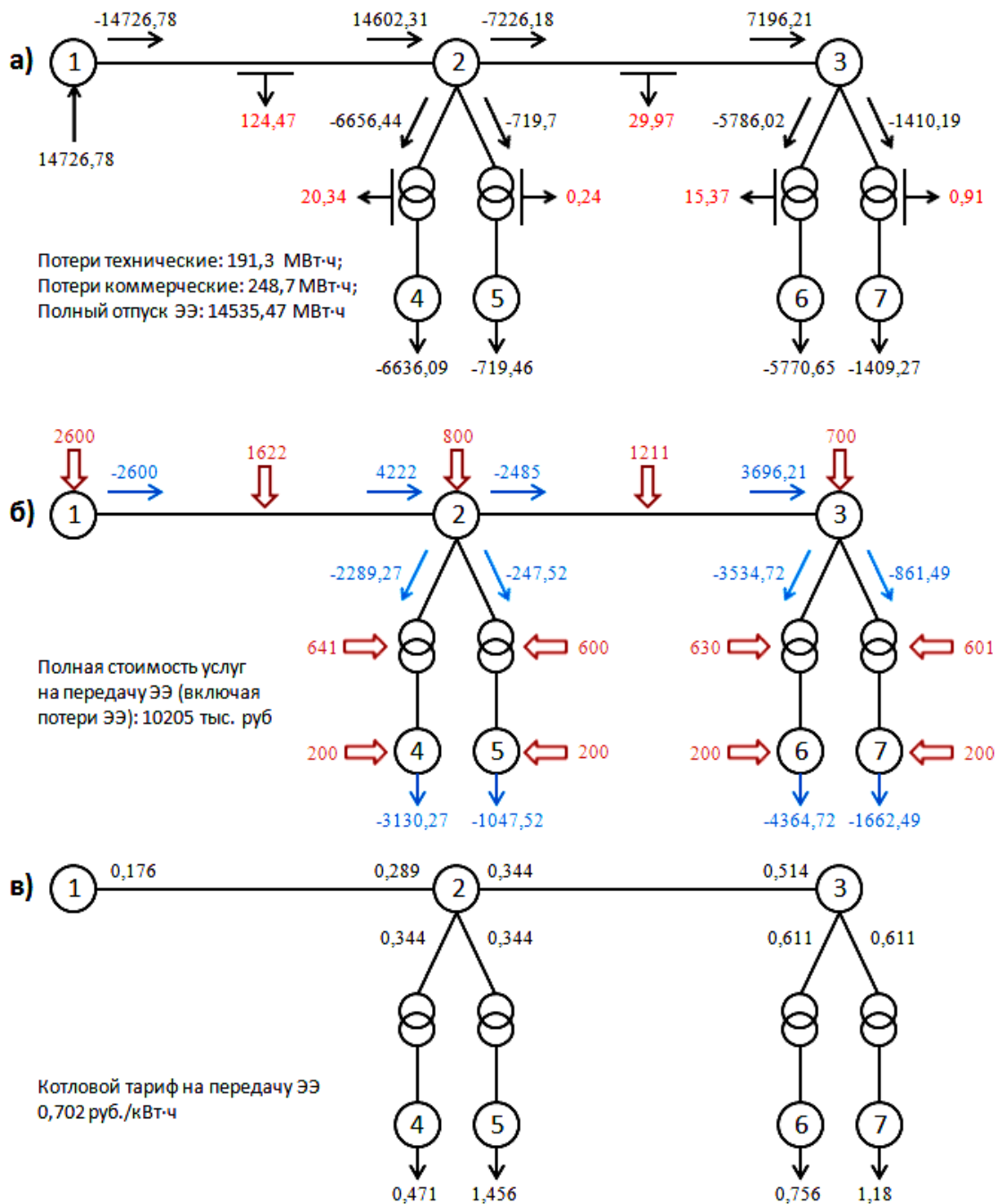
Рисунок 5. Распределение на схеме электрической сети:
