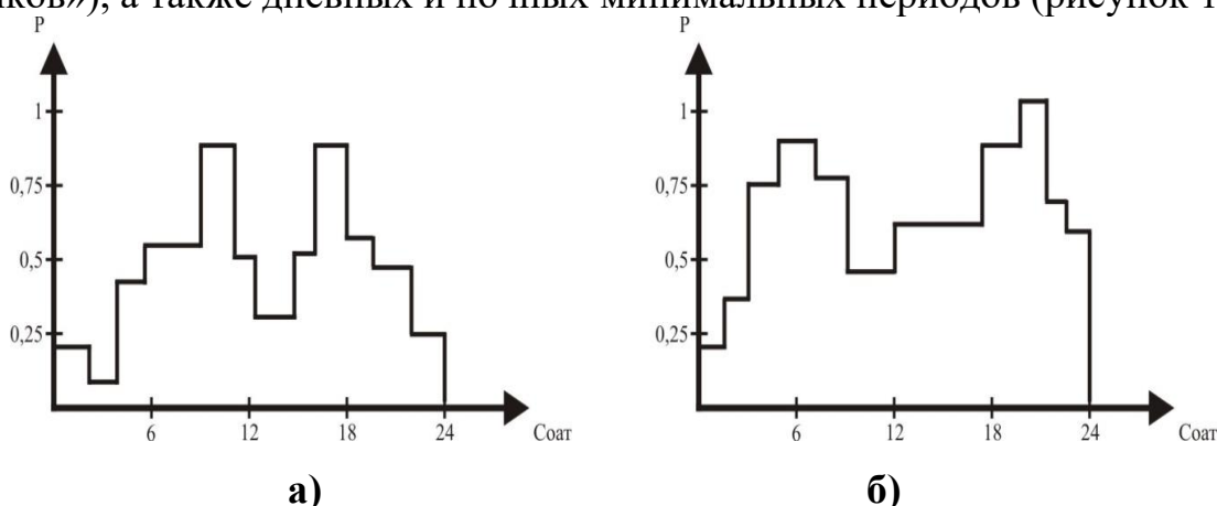
Рисунок 148. В зимний (а) и летний (б) сезоны подстанции изменения графиков электрических нагрузок
