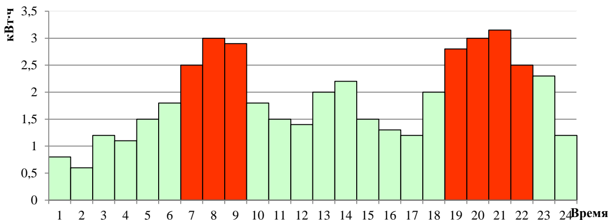
Рисунок 150. Суточное потребление электрической энергии населением в рабочие дни
