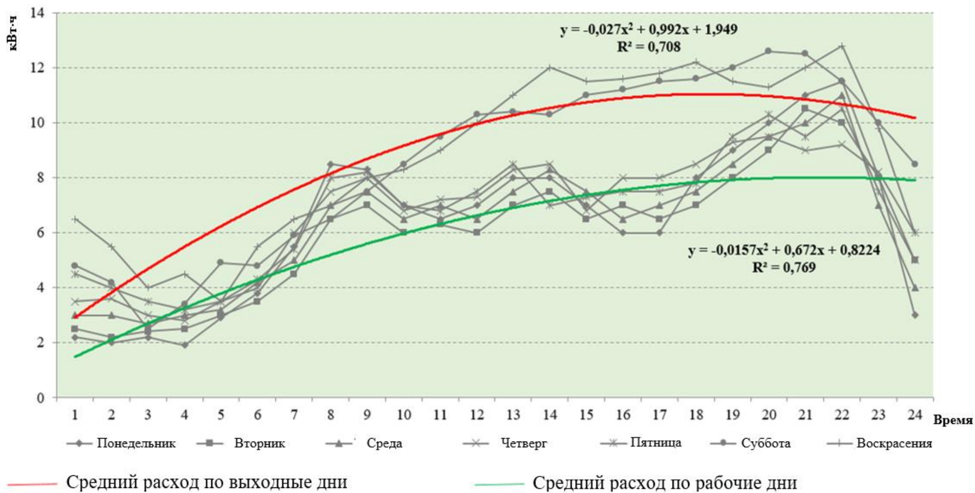
Рисунок 156. Графики почасового изменения потребления электрической энергии в мае 2019 года населением Мирабадского района (месяц минимального потребления электрической энергии в году)
