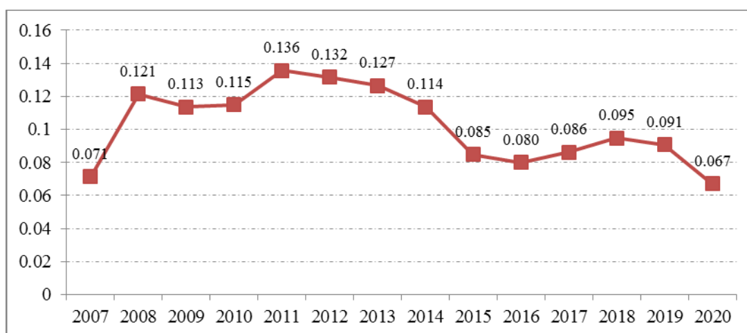
Рисунок 49. Тарифы на электроэнергию, поставляемую от ТЭЦ-1, за период 2007-2020, $/кВт*ч
