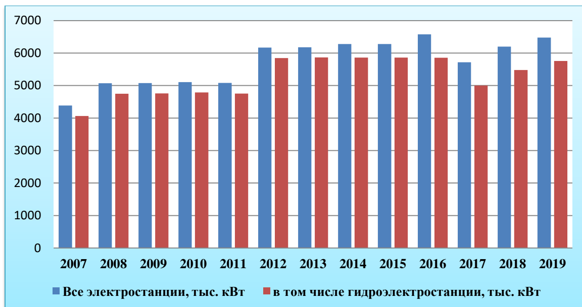
Рисунок 24. Установленная мощность электростанций в 2007-2019 гг., тыс. кВт
