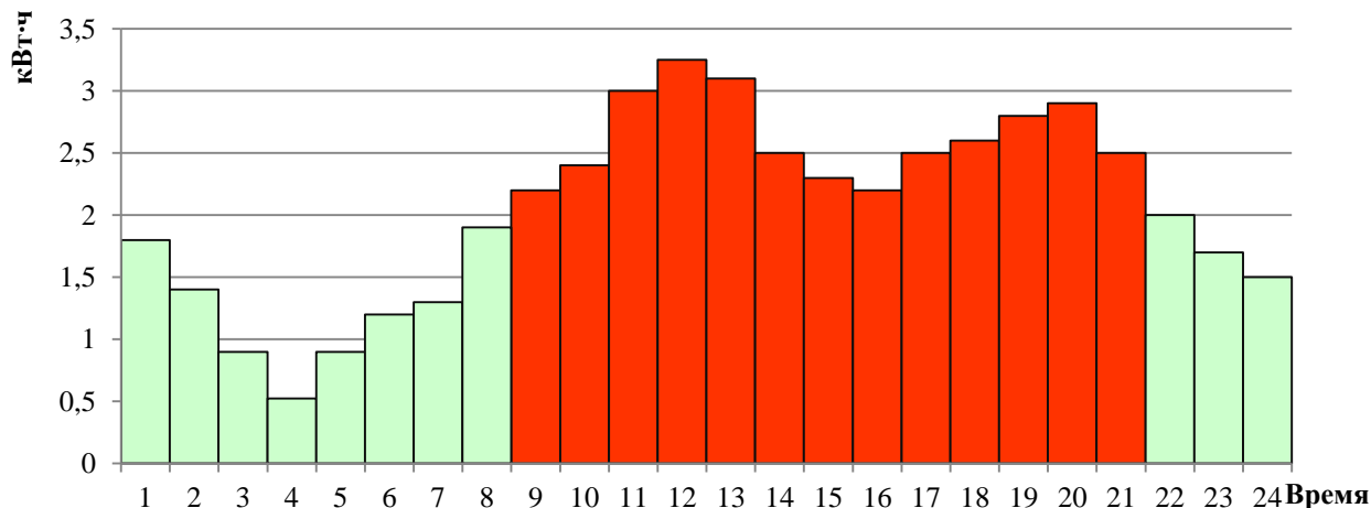
Рисунок 151. Суточное потребление электрической энергии населением в выходные дни.
