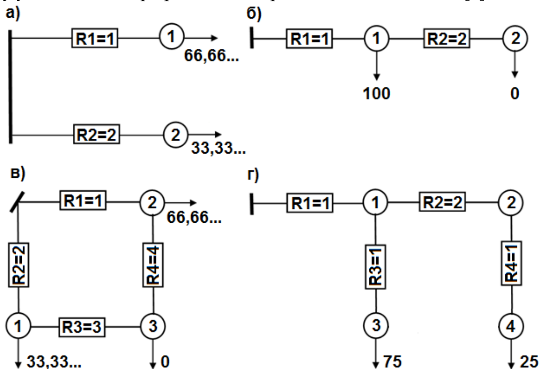
Рисунок 6. Распределение в электрической сети оптимальных мощностей, полученных по критерию равенства ОППМ, при различных вариантах топологии.
