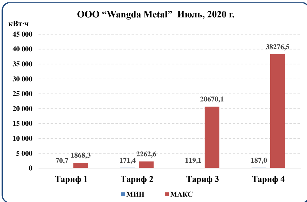
Рисунок 38. Максимальное и минимальное потребление электроэнергии в ООО Wangda Metal в июле 2020 г.
